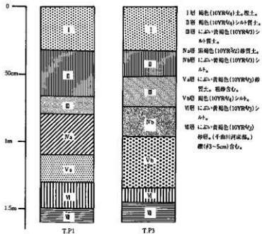
基本土層模式図
