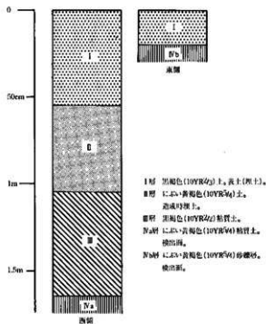
基本土層横式図
