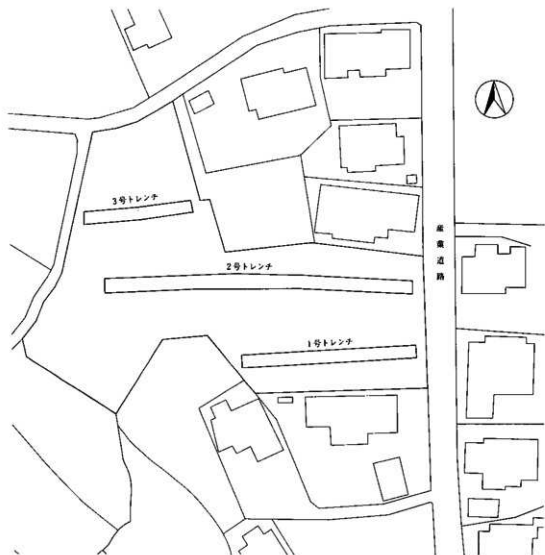
試掘トレンチ設定図 (1 : 800)
