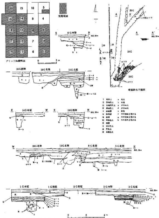
第5図 下の丁地緯平面・断面図
