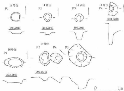
図105 14・16号住柱穴実測図
