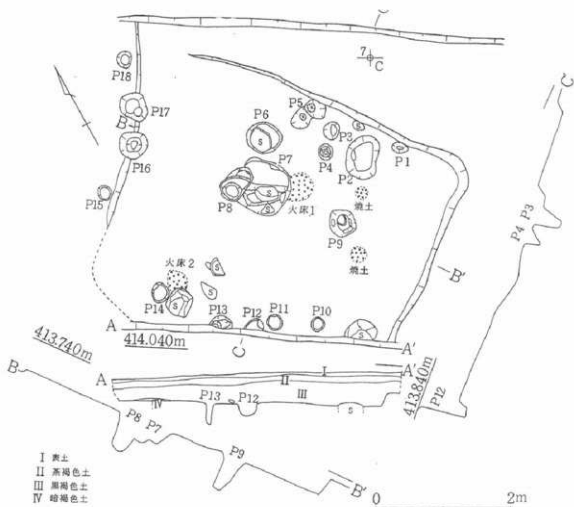
図74 51号住遺構実測図
