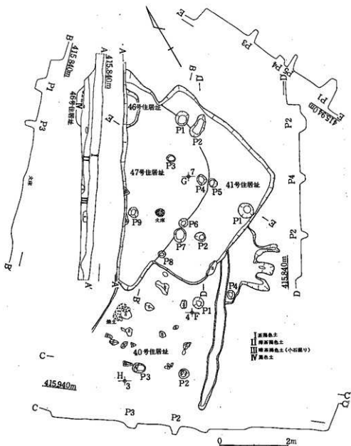
図48 40・41・46・47号住遺構実測図
