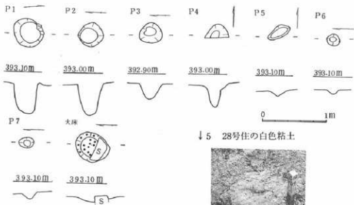
図17 28号住柱穴実測図
