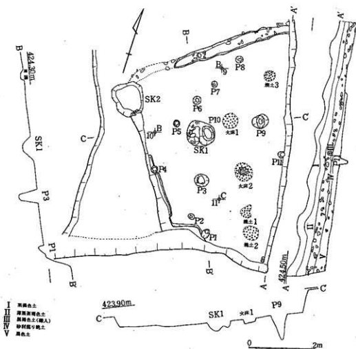
図22 31号住遺構実測図
