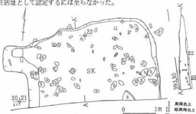
図5 支線1号縄文土坑実測図
