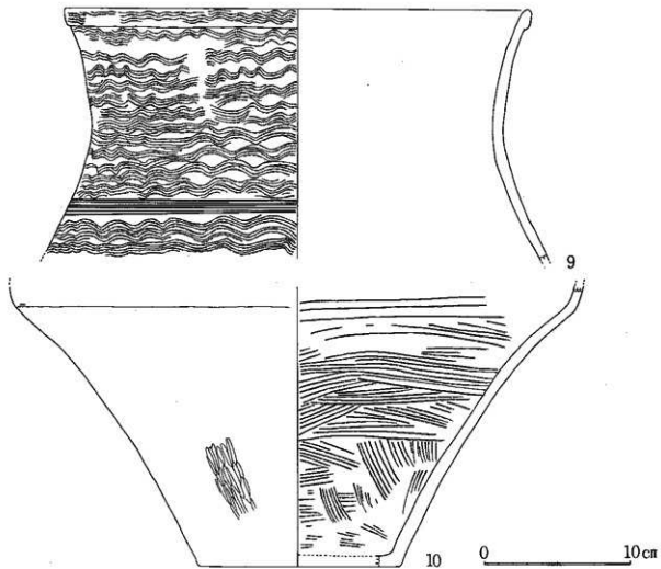
图68 48号住出土土器実測図(2)
