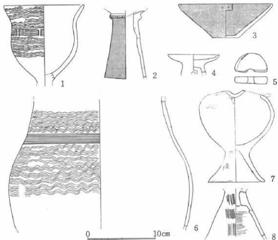
図42 39号住出土土器実測図
