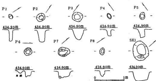
図129 34号住柱穴・土坑実測図
