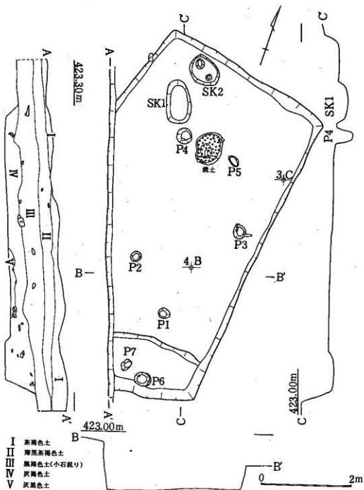
図116 32号住遺構実測図
