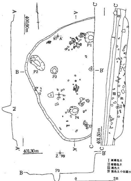
図111 27号住遺物・遺構検出実測図
