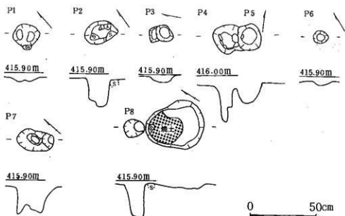
图40 39号住柱穴・烧土实测图
