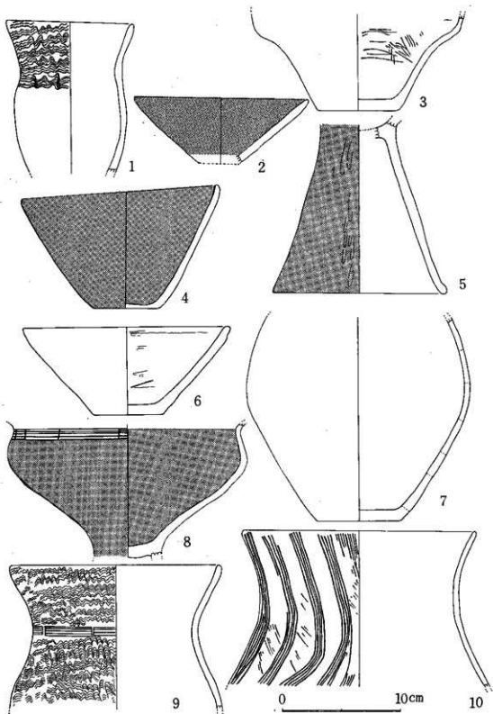
图75 51号住出土土器实测图(1)
