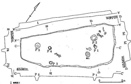
図61 45号住遺構実測図
