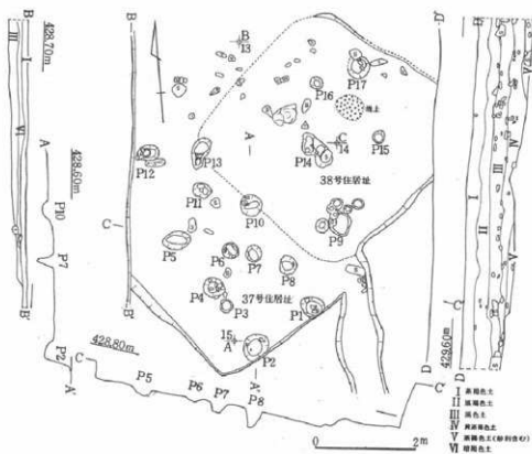
図36 37・38号住遺構実測図
