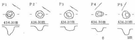
図124 33号住柱穴実測図
