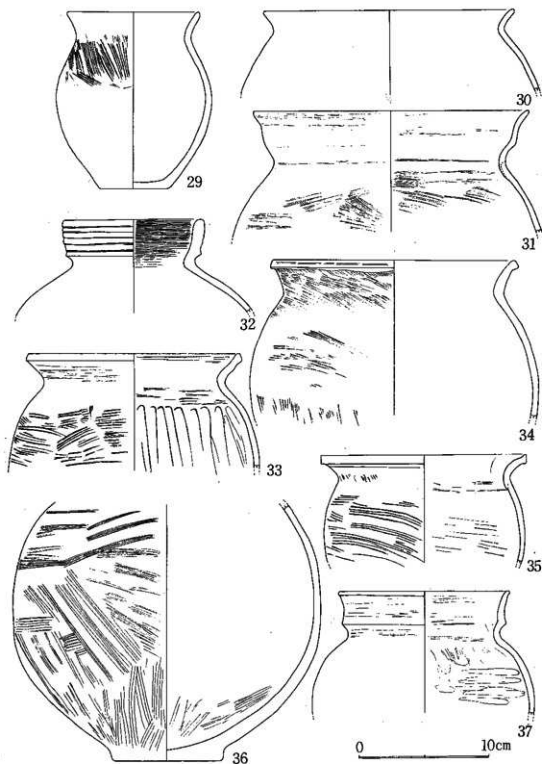
图120 32号住出土土器实测图(3)
