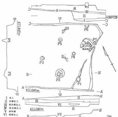
図131 49号住遺構実測図
