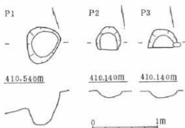
図65 48号住柱穴実測図
