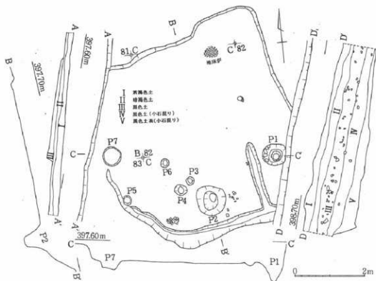
図110 20号住遺構実測図
