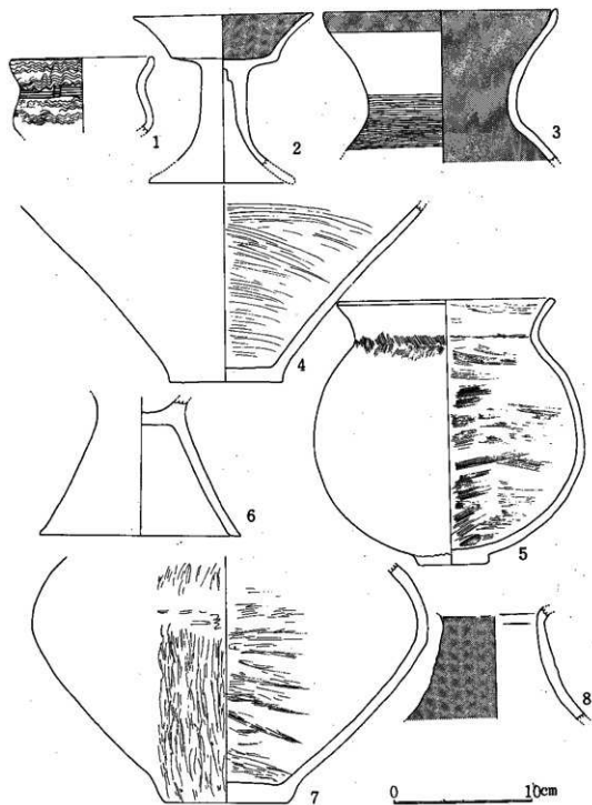
图16 土器实测图（支線1号 28・29・30号住）
