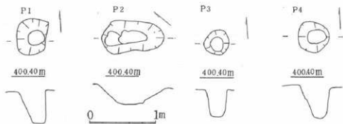
図112 27号住柱穴実測図
