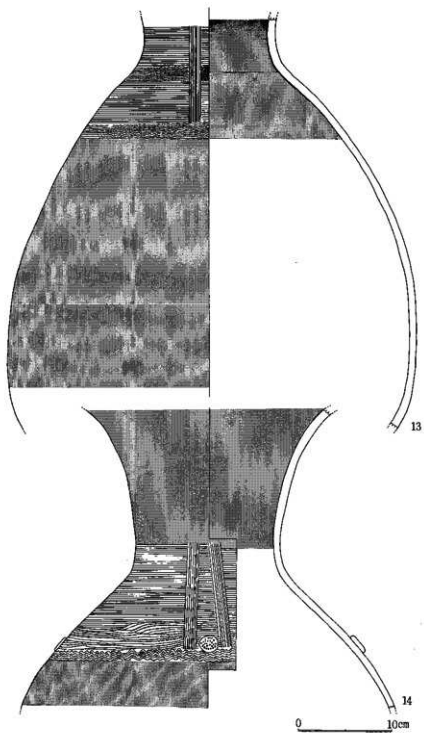
图60 45号住出土土器实测图(3)
