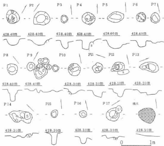
図37 37・38号住柱穴・焼土実測図
