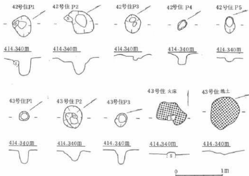
図53 42・43号住柱穴・焼土実測図
