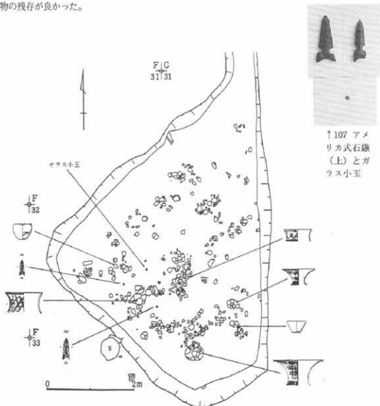
図145 6号住遺物出土実測図
