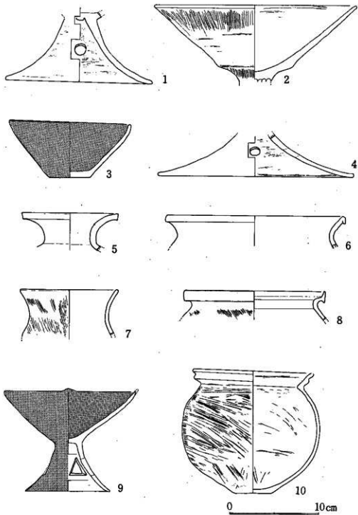
图94 7号住出土土器实测图(1)
