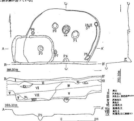
図15 28号住遺構実測図
