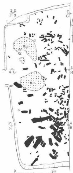
図91 7号住遺物(炭)実測図
