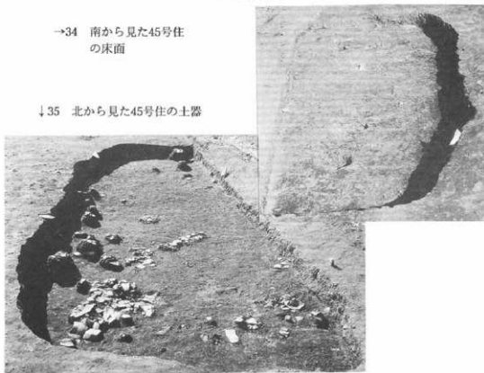
図57 45号住遺物検出図
