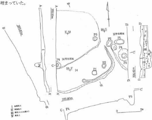
図101 14・16号住遺構実測図
