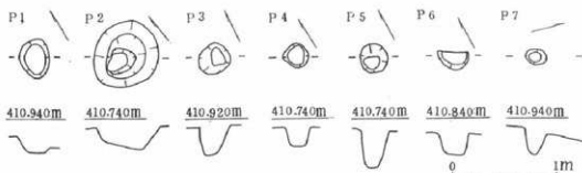
図134 49号住柱穴実測図
