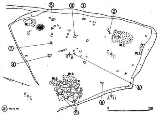
図21 31号住遺物検出図
