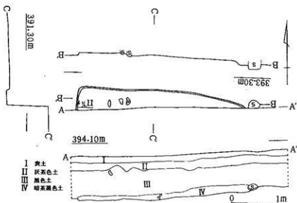
図20 29号住遺構実測図
