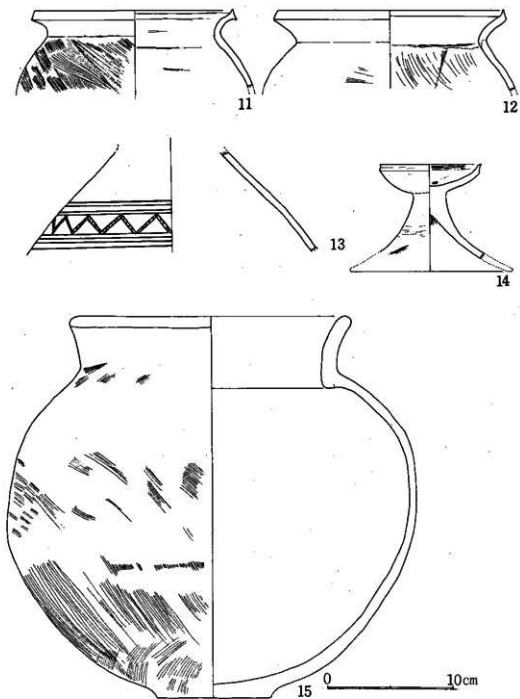
图95 7号住出土土器实测图(2)
