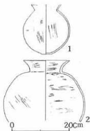
図104 14号住出土土器実測図
