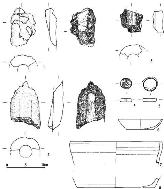
第8図 第1号製鉄炉址出土遺物実測図(1:3)
