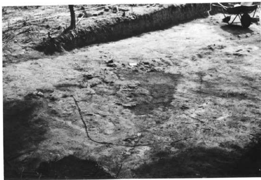
第1号製鉄炉址（炉底部）
