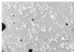
新潟県北蒲原郡豊浦村奥木山 (平安末期頃の原始的製鉄所) 共品質の中に懸濁した細かいマグネタイト
