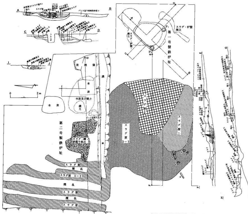
第7図 第一号製鉄炉址及び第二号製鉄炉址平面図
