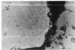
(ウイドマンスラッシュ) ×500
