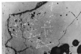
E 坂城町開設2号が跡鉄棒E×100
