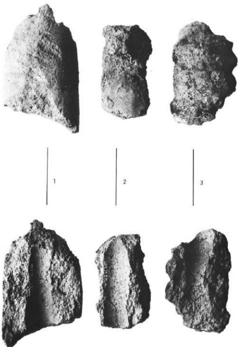
第1号製鉄炉址出土の遺物①(1~3羽口片)
