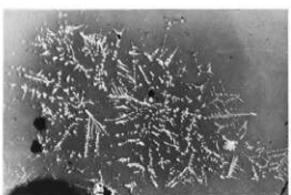
D 1号炉跡鉄滓D×100
