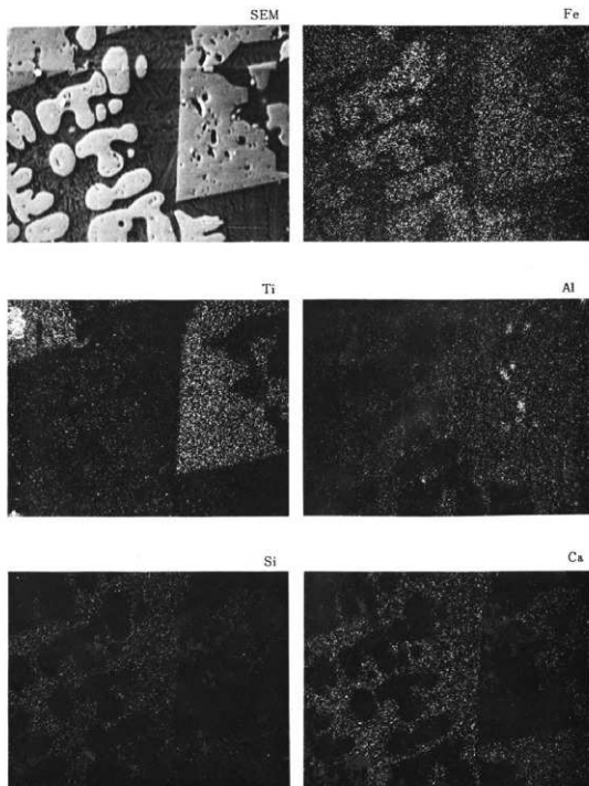
間鉄製鉄遺跡鉄滓(第1次図版11)のマイクロアナライザーによる分析①
