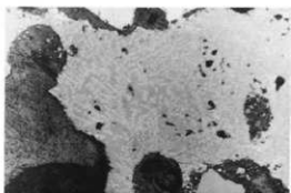
B 1号炉跡鉄滓胎状鉄滓B×100
