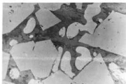
A 板城町開設1号炉跡胎状鉄滓C×100
