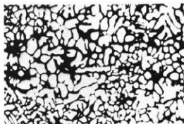
滋賀県埴内遺跡鍛冶埴 (鎌倉期頃の鍛冶工房に伴うもの) 白い丸状の部分がウースタイト
