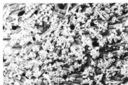
雪花状はマグネタイト 熊本県玉名市春日久段製鉄遺跡 (鎌倉期頃の原始的製鉄炉)
