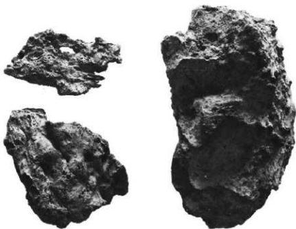
鉄滓 (左: 海綿状鉄滓、右: アメ状鉄滓)
