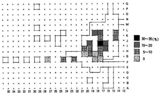
第10図 炉壁破片の分布
