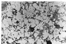
A 1号炉跡やや粗雑な鉄滓A×100
