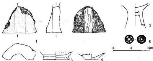
第9図 第2号製鉄炉出土遺物実測図(1:3)
