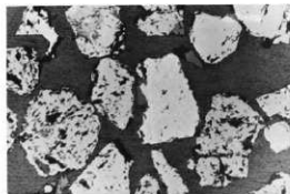
ピット内探集砂鉄×100
