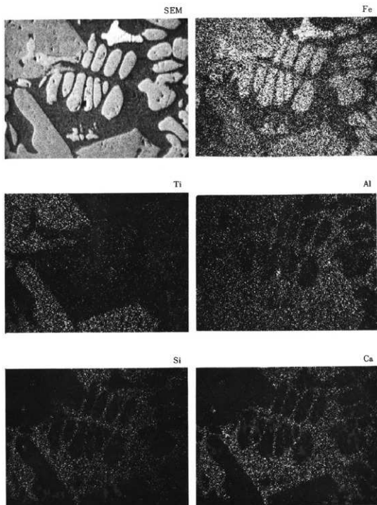
開飲製鉄遺跡鉄滓(第1次図版11)のマイクロアナライザーによる分析②
