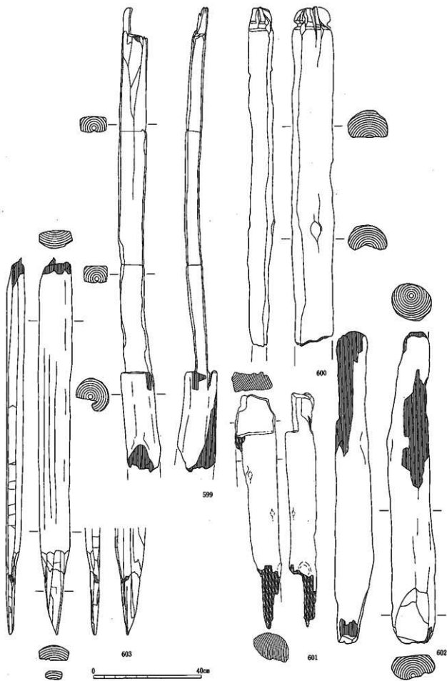
建築部材 柱(599~603)
