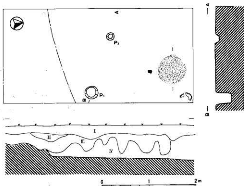
第4図 F-22 検出遺構 (1:40)
