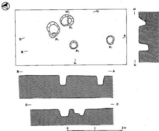
第10図 O-7検出遺構(1:40)
