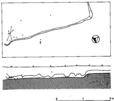
第6図 E-3 検出遺構 (1:40)
