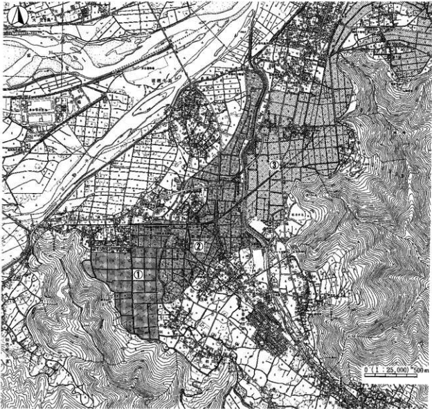
第13図 若穂川周辺の水利ブロック
