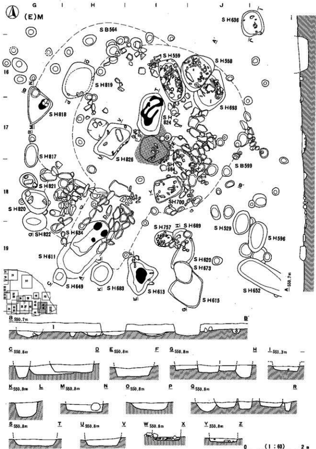
土層 1: 礫を含む黒褐色粘質土、骨片・炭化物混在 2: 暗褐色粘質土 3: 黒褐色粘質土 4: 赤褐色粘質土、炭化物多量に混在 5: 赤褐色ブロックを含む暗褐色粘質土、炭化物混在 6: 赤褐色土粒を含む黒褐色粘質土、炭化物混在
