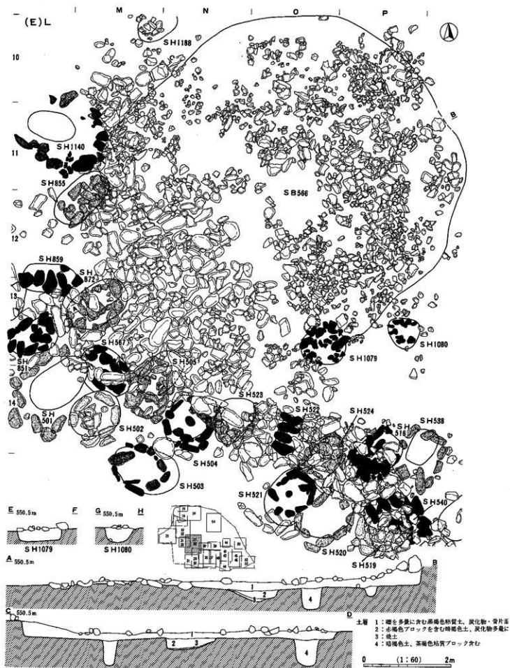
図版27 縄文遺構図17 (SB566, SH501ほか)
