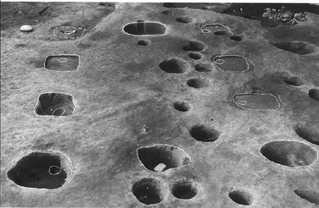
403号建物跡 (東より)
