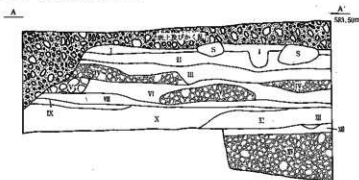
第6図 伊勢町27次3面第1号建物址
