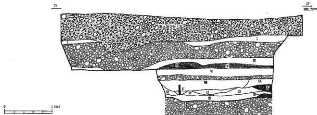
第8図 伊勢町28次土層図
