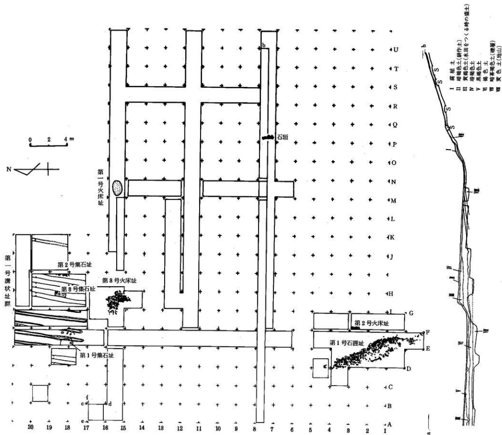
第7图 開成製鉄遺跡平面図
