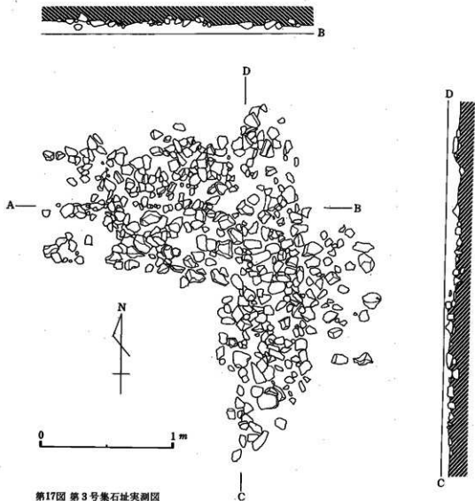
第17図 第3号集石址実測図
