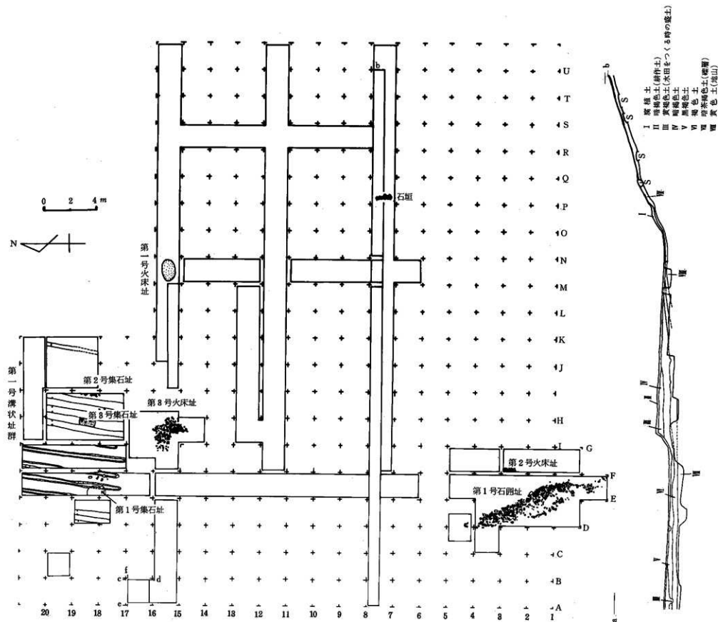
第7图 開飲製鉄遺跡平面図
