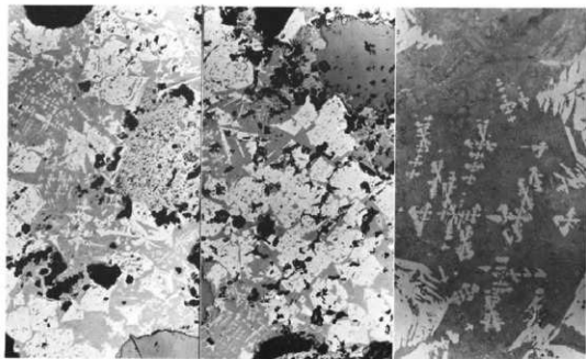
B：坂城町間蔵遺跡の鉄滓（多孔酸化鉄状のもの）
