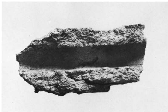
羽口 (P-12グリッド)
