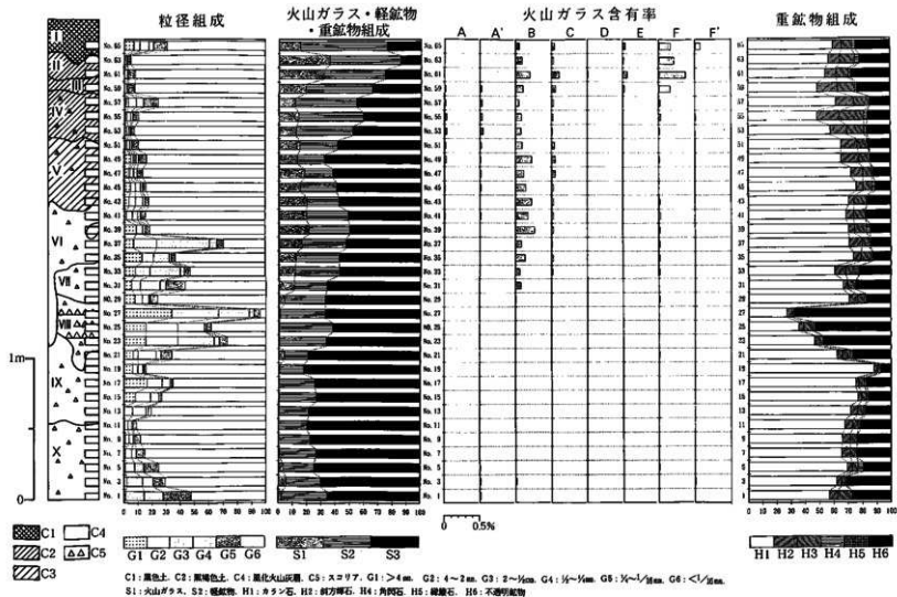
第15図 関山遺跡の柱状図、粒径組成、火山ガラス・軽鉱物・重鉱物組成、火山ガラス含有率、および重鉱物組成
