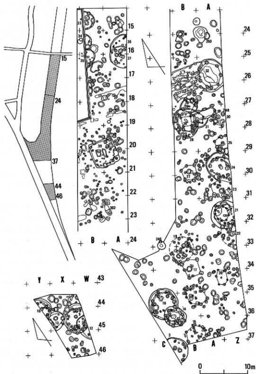
甲ッ原遺跡 全体図 (1/400)
