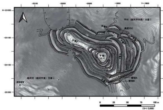
第4図 西屋敷小屋館跡 縄張り図
