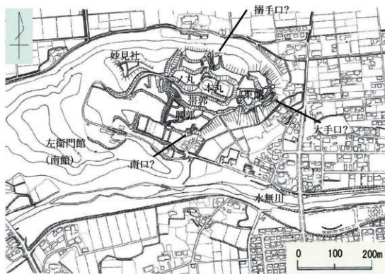
図4 牛越城縄張図
