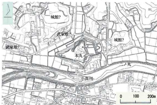
図2 小高城縄張図
