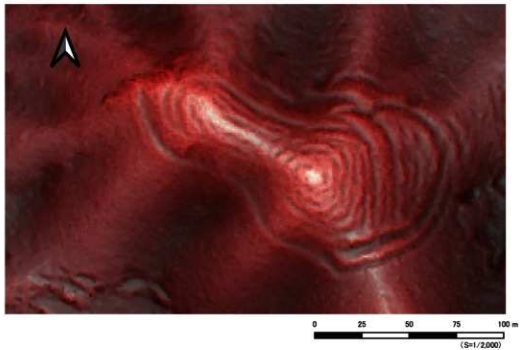
第3図 西屋敷小屋館跡 赤色立体地図
