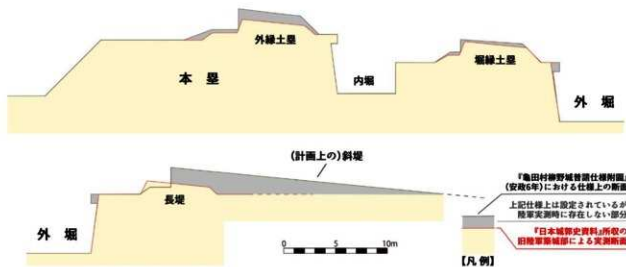
図 52. 『龜田村柳野城普請仕様附圖』（安政 6 年）および『日本築城史資料』（大正～戦前）における五稜郭の壁・壕（堀）断面図の比較
