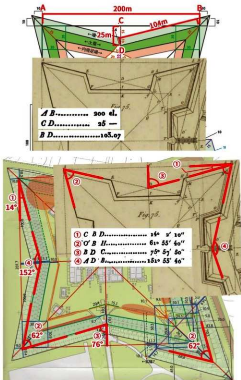
図 41. サヴァール教本において示された標準的な稜堡式要塞設計の具体的数値と、戸切地陣屋との寸法（上）および角度（下）における一致
