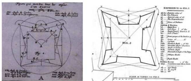
図 34. 伝ヴォーバン教本 (1695 年版本、図左) およびストレイス教本 (1852 版本、図右) に見られる、正方形を基準とする四稜堡構造の模式図
