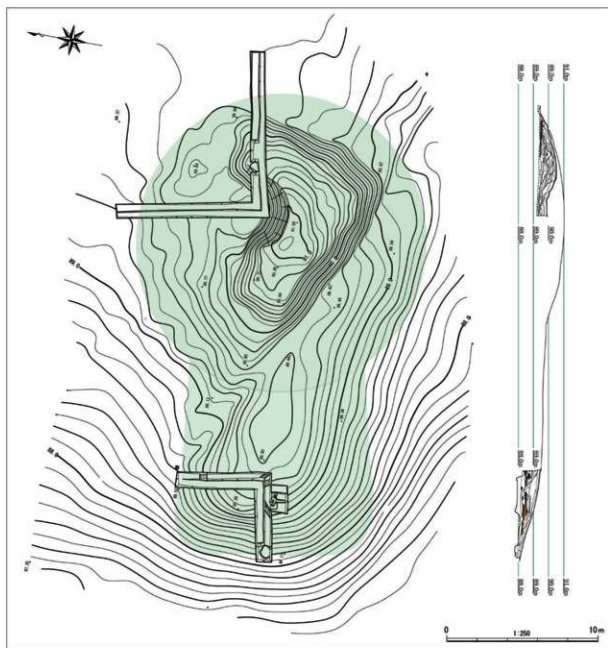
図4-3 杉洞1号墳墳丘復元図
