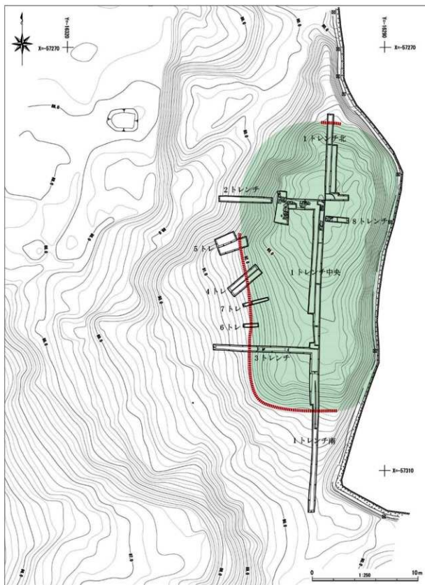
図4-2 蓮野1号墳墳丘復元図
