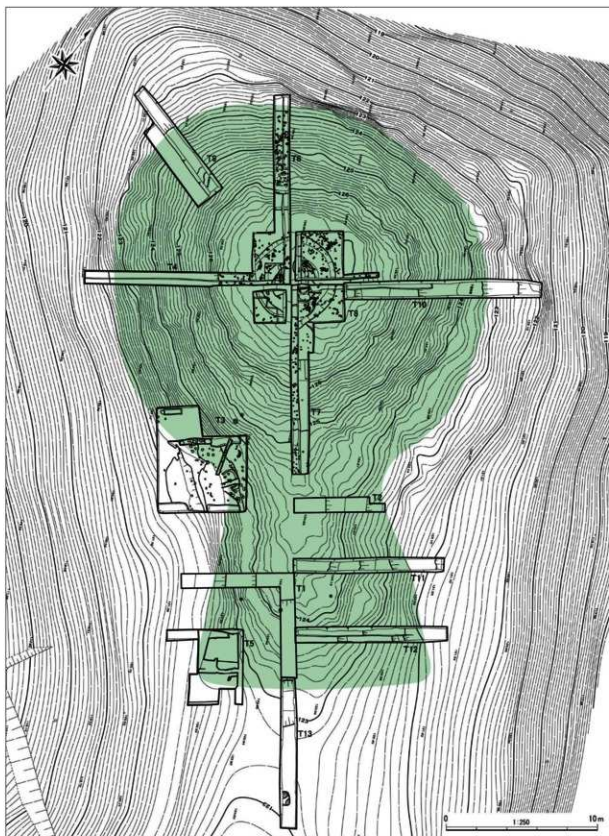
図4-1 夕田茶臼山古墳墳丘復元図
