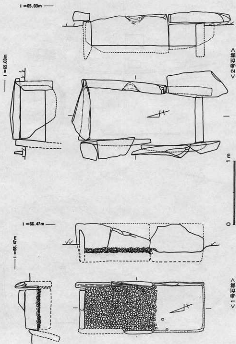
(第4図 久井原埴城塔石棺実測図)
