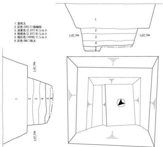
図2 調査区平面・土層断面図
