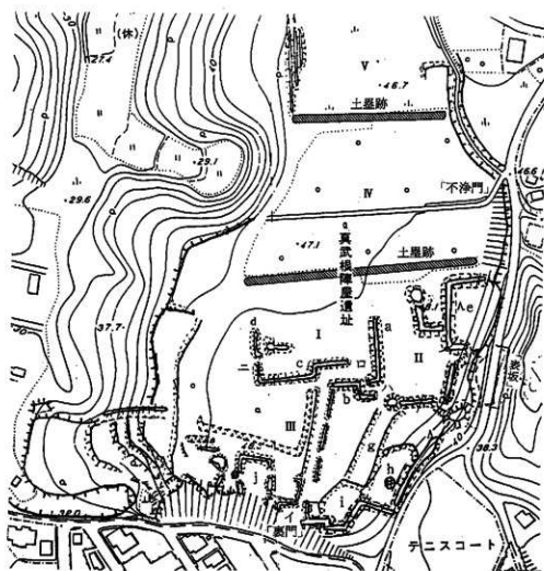
真武根陣屋跡概念図 (松本勝・矢野淳一・稲垣昭智原図に加筆)
