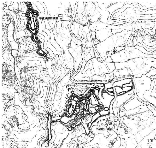
第1図 平蔵城跡配置図
