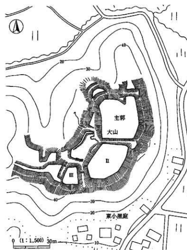
日在城跡概念図
