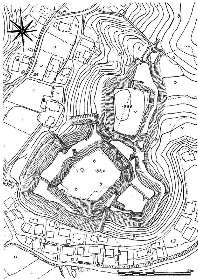
大倉城跡概念図
