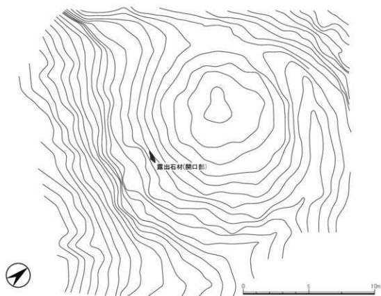
図3 8号墳測量図
