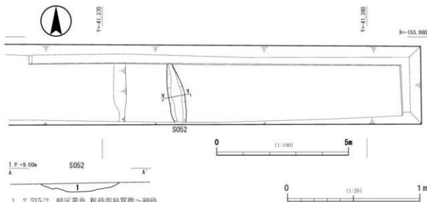
図 28 8区第2面部分平面・遺構断面
