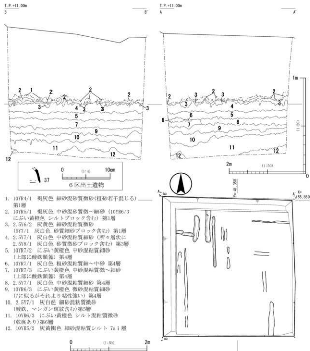
図17 6区平面・土層断面
