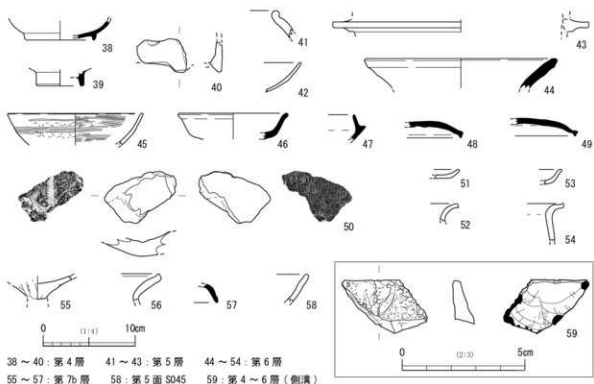
図 24 7 区出土遺物実測
