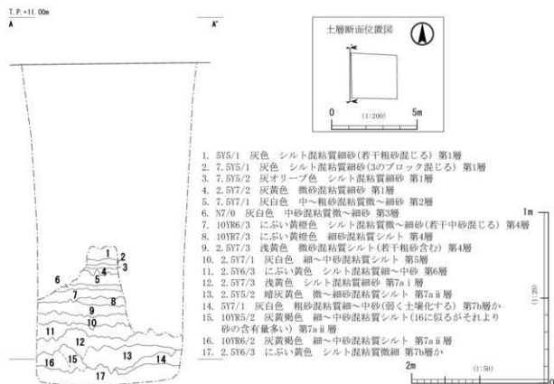
図9 3区土層断面
