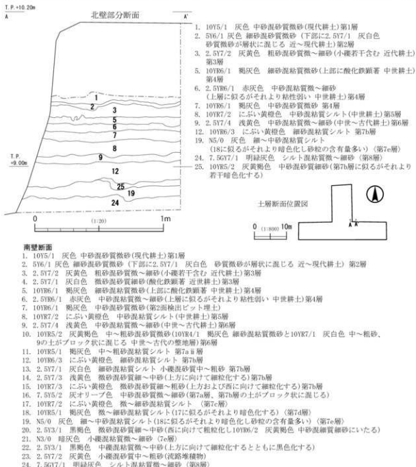
図 19 7 区北壁部分土層断面等
