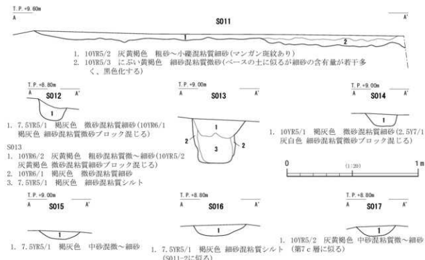
図15 5区遺構断面
