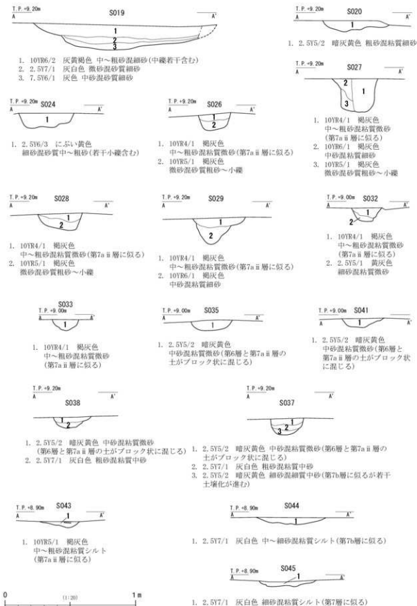
図 23 7 区遺構断面
