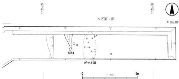
図 25 8区・9区平面等
