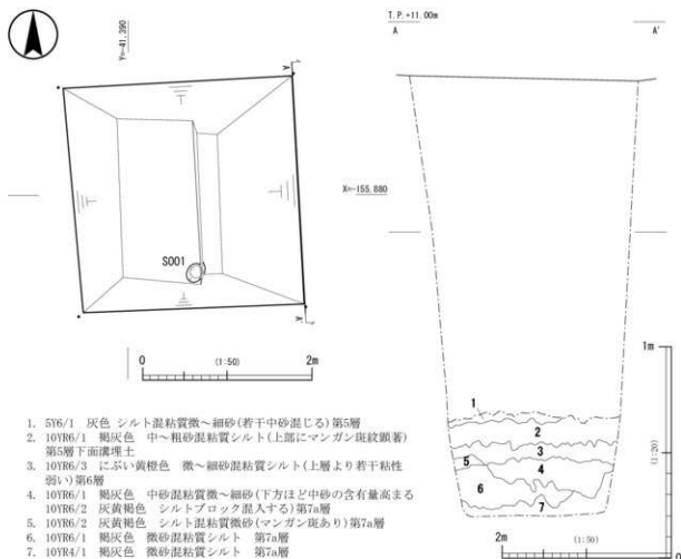
図7 1区平面・土層断面
