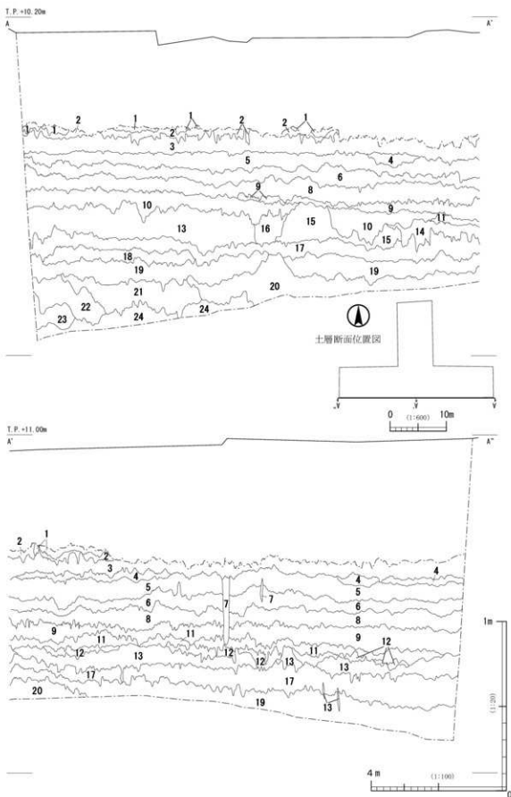
图 18 7 区南壁土层断面
