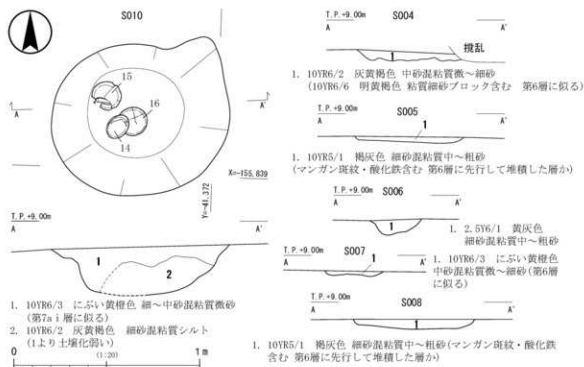
図13 5区遺構平面・断面
