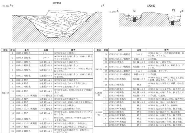
第16図 SA2633 柱列跡・SD2150 溝跡断面図
