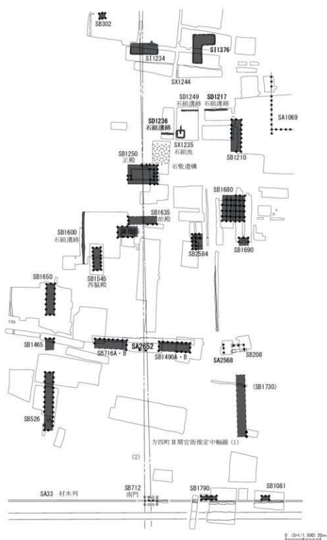
第8図 方四町Ⅱ期官衙中核部主要遺構配置図
