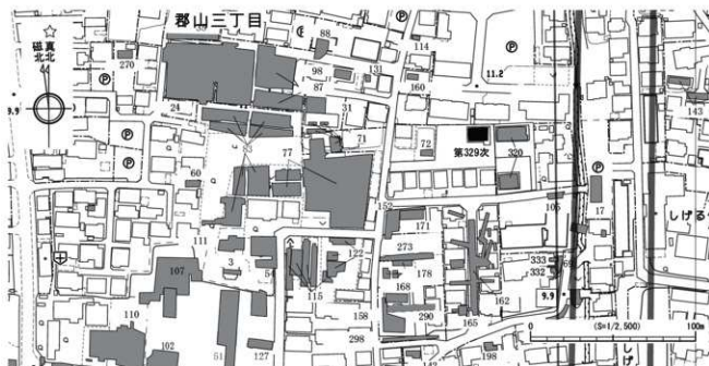
第10図 第329次調査区位置図
