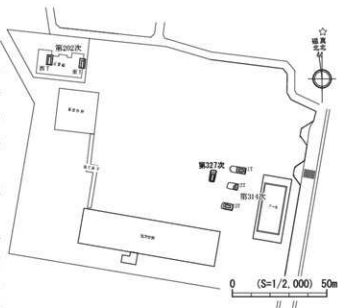
第26図 第327次調査区配置図
