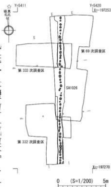
第22図 第332・333次調査 遺構配置図
