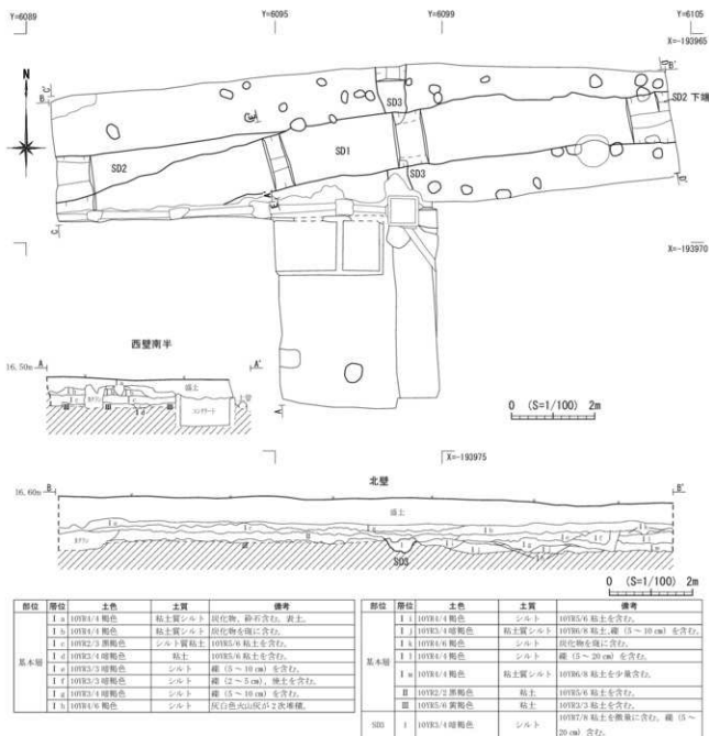
第32図 第33次調査 1区平面・断面図
