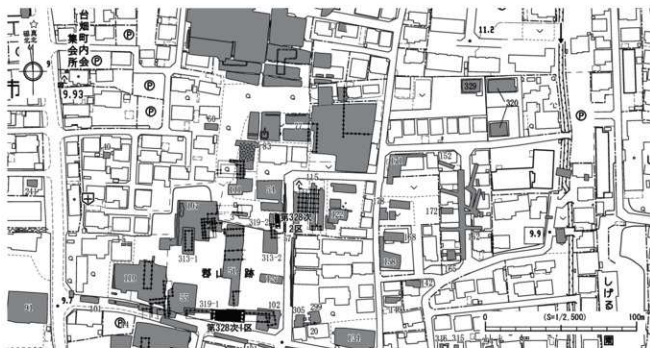
第3図 第328次調査区位置図
