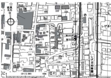
第21図 第332・333次調査区位置図
