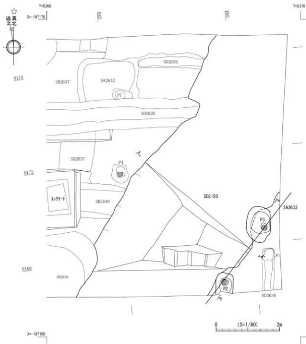
第15図 SA2633柱列跡・SD2150溝跡平面図
