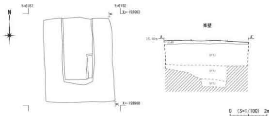
第39図 第33次調査 4区平面・断面図
