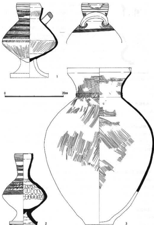
图37 遗物实测图 (1/4)
