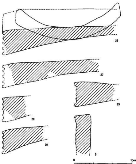
図15 軒瓦実測図 (1/3)
