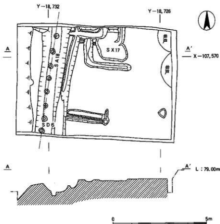
図25 遺構実測図 (1/100)
