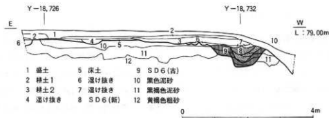
図26 南壁断面実測図 (1/80)
