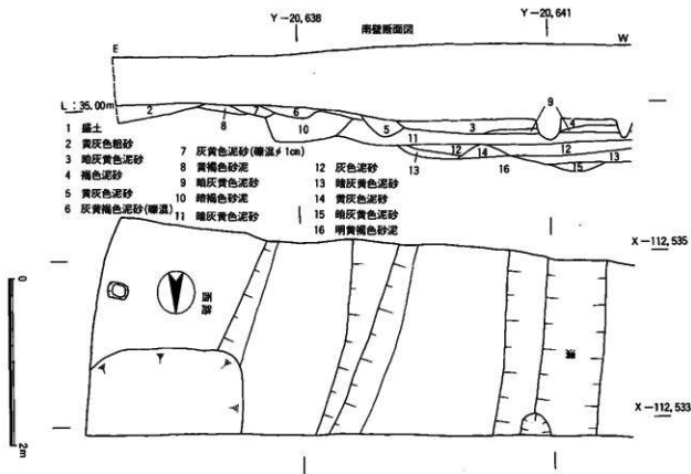
图30 崖横断面图 (1/50)
