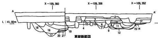
東壁断面図
