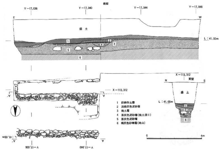
图33 遺構実測図 (1/80)
