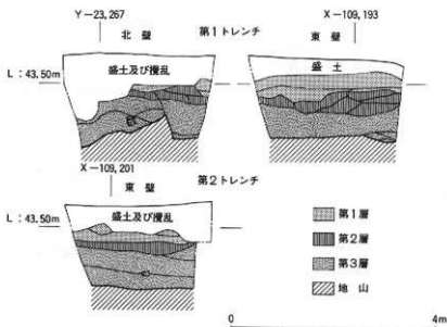
図3 断面実測図 (1/80)
