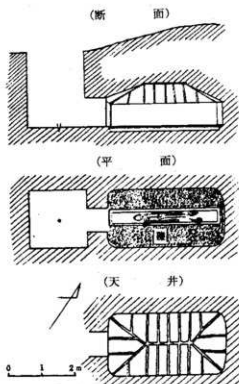
六野原地下式第2号墳実測図(「六野原古墳調査報告書」による)
