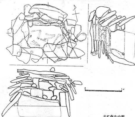
第31図 浜郷遺跡(第二次) 1号石棺構造図
