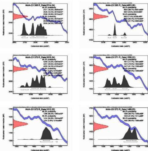
図1 暦年較正年代グラフ
