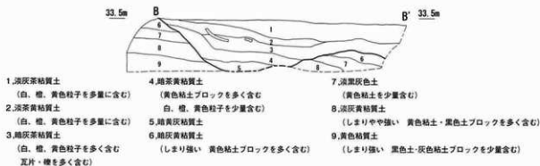
第61図 南北方向版築状遺構土層図 (1/30)
