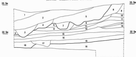
第60図 1トレンチ南壁土層図 (1/30)
