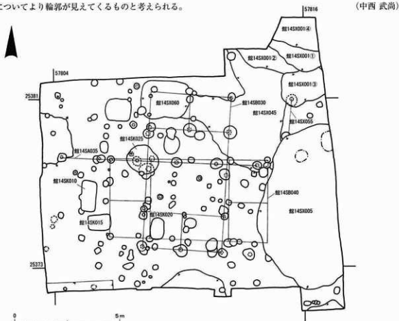
第7図 第14次調査区遺構配置図 (1/125)
