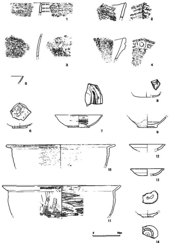
第90図 出土遺物実測図 (1/4)
