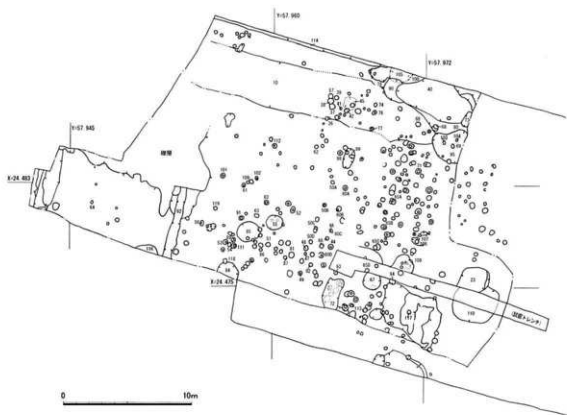
第29図 遺構配置図 (S=1/200)
