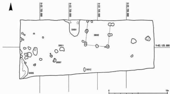
第99図 遺構略測図 (1/200)
