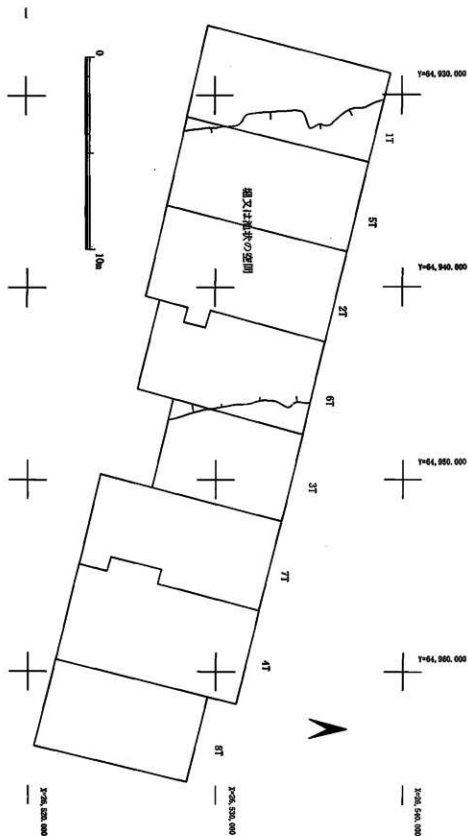
第105図 鶴崎町遺跡群(堀川)遺構配置図(1/200)
