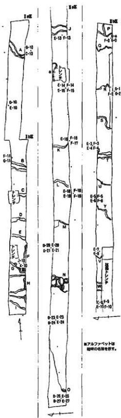
第65図 Ⅱ・Ⅲ調査区第3号水田遺構配置図(S=1/300)
