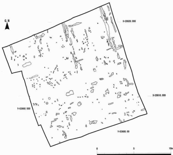
第102図 S003水田層遺構配置図(1/150)
