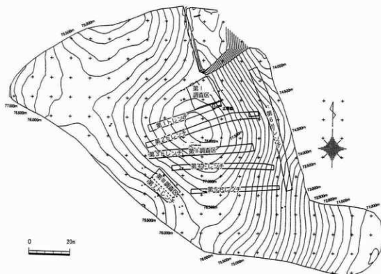
第48図 調査区・試掘トレンチ位置図 (1/1250)
