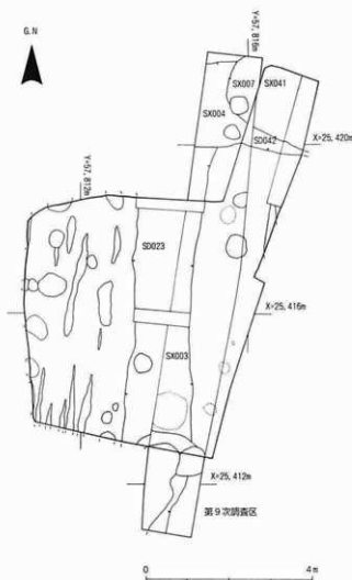
第33図 A地点 遺構配置図（1/100）
