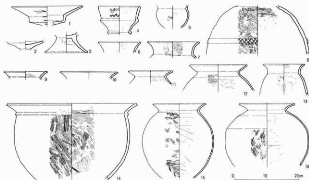
第26図 SX002出土遺物実測図 (1/6)
