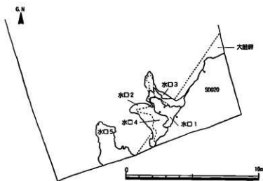
第75図 水口遺構配置図（1/200）
