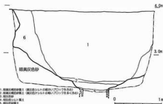
第70図 SE006土層断面図（1/40）
