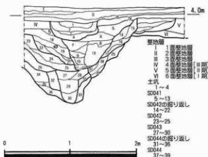
第34図 A地点東西溝土層断面図（1/40）
