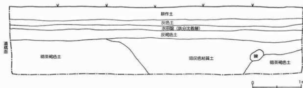
第103図 第4トレンチ南壁土層断面図（1/40）
