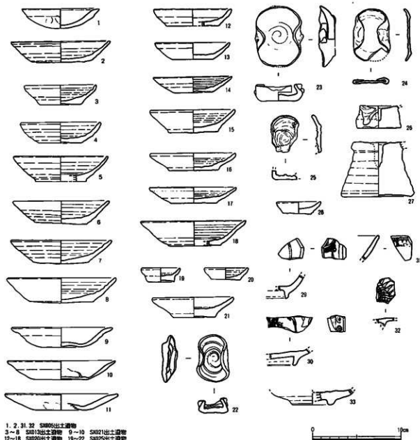
第46図 出土遺物 (1/3)
