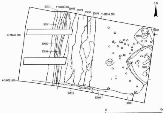
第11図 遺構配置図 (1/200)
