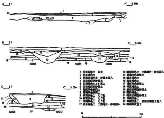
第44図 調査区南壁土層図 (1/40)
