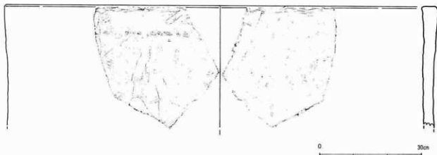
第56図 SE270出土土師質井戸枠実測図 (1/8)
