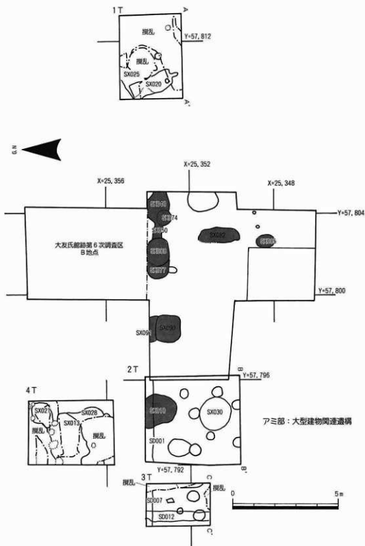
第43図 遺構配置図 (1/125)
