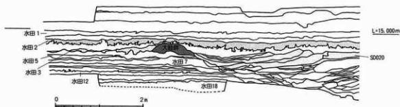
第77図 調査区南側東壁土層断面図(1/60)
