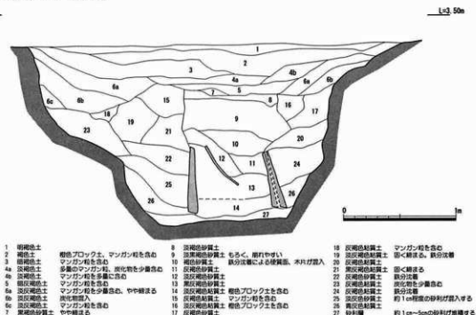
第94図 SE002土層断面図(1/30)
