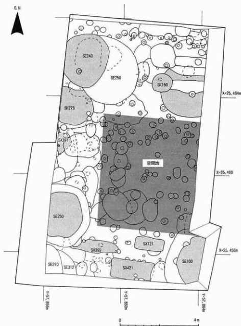
第53図 遺構配置図 (1/100)
