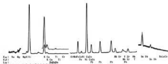
図4 秋月遺跡出土青ガラス玉 985-29(108428)の蛍光X線スペクトル
