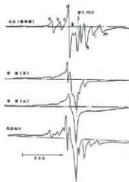
図5-3 碧玉原石の信号 (Ⅱ) の ESR スペクトル
