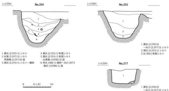
図8 古墳時代前期の遺構 断面図
