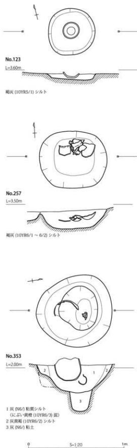
図 28 古代の遺構 遺物出土状況図
