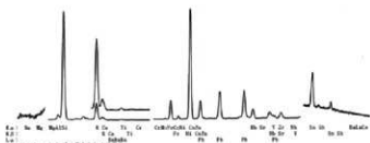
図3 秋月遺跡出土青ガラス玉 1160-28(108427)の蛍光X線スペクトル
