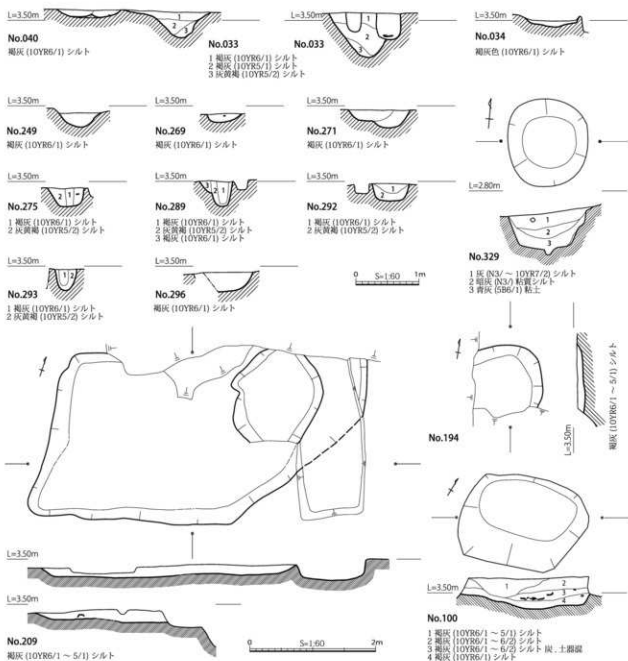
図 27 古代の遺構 (北半) 平面図・断面図
