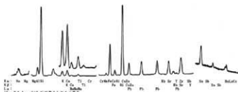
図2 秋月遺跡出土青ガラス玉 1160-27(108426)の蛍光X線スペクトル
