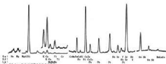
図6 秋月遺跡出土赤ガラス玉 985-31(108429)の蛍光X線スペクトル
