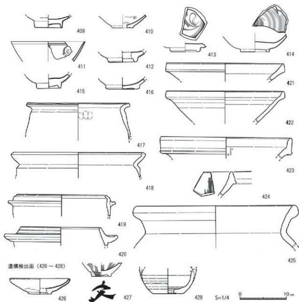
図 64 001 大土坑出土土器実測図②(陶磁器)
