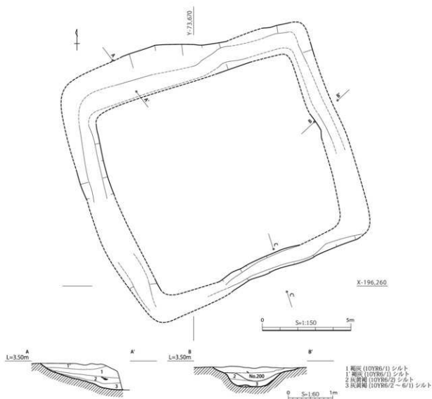
図 20 秋月 12 号墳 平面図・断面図
