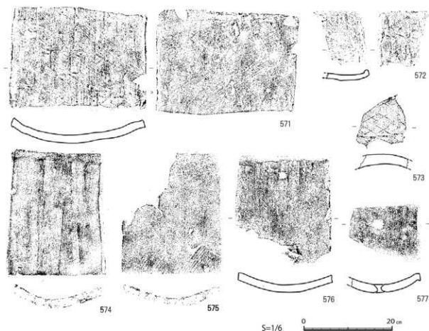
図 75 平瓦実測図
