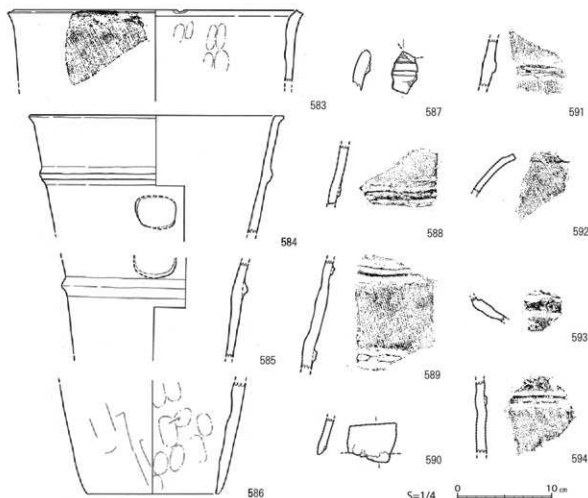
図77 埴輪実測図
