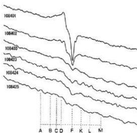
図6 秋月遺跡出土碧玉の ESR 信号 (Ⅲ) のスペクトル
