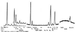
図 3-6 秋月遺跡緑色凝灰岩製管玉 965-23(108425)の蛍光 X 線スペクトル
