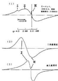
図4 碧玉原石の ESR スペクトル (花仙山、玉谷、横八、土岐)
