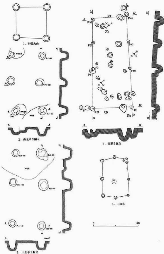
第2図 竪立柱建物址 (S=1/100)
