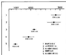
図-8 開闢岳活動開始時期の 14 C年代
