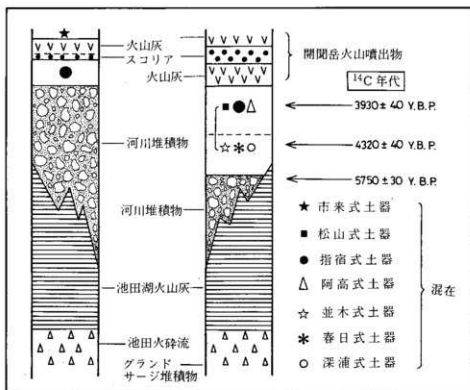
↑ 図-6 田中遺跡と成川遺跡地質柱状図
