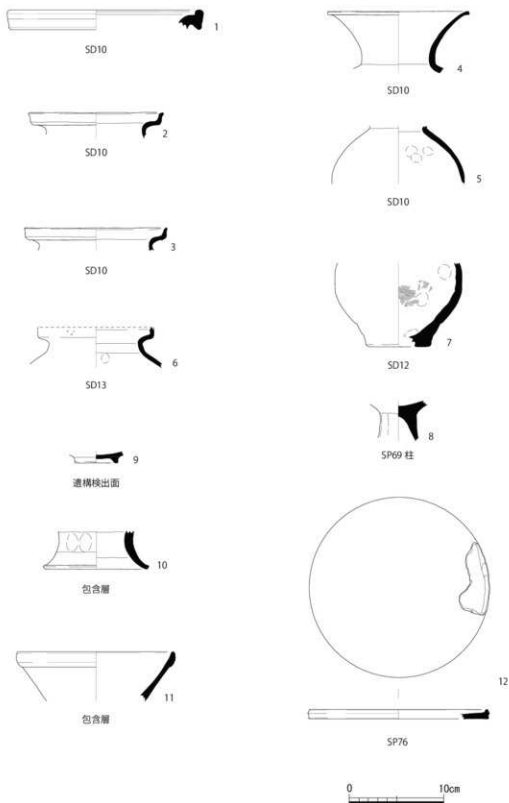
第3図 出土遺物実測図
