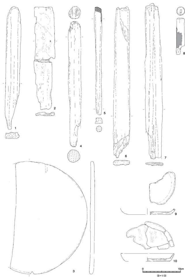
第19図 1区 SK03、SK07、SD07、SD08出土遺物 (S = 1/3、1/6)
