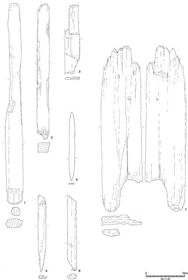
第20図 1区 SD08、SD07・08、2区 SK04出土遺物 (S=1/3)
