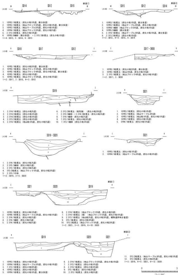
第10図 2区 SD12・SD14・SD15、SD12・SD17・SD18、SK08・SD17、SD19、SD21、SD19・SD20、SD21、SD19・SD20・SD21 (S=1/60)
