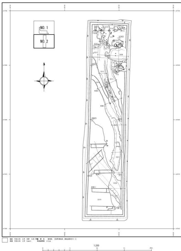
第7图 2区 遺構全体図 (S=1/200)
