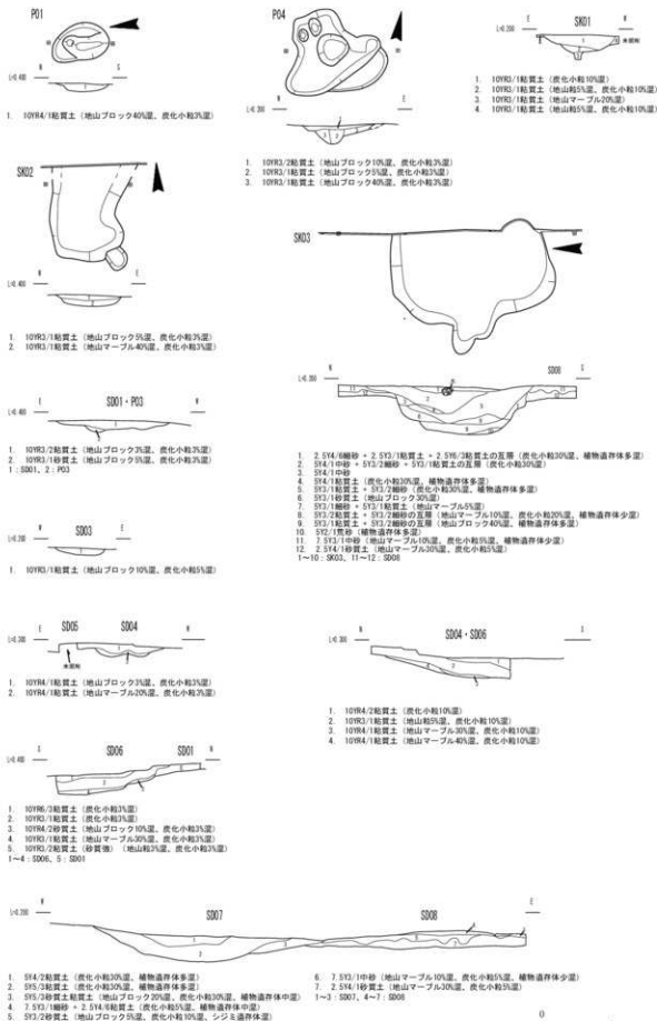
第8図 1区 P01、P04、SK01、SK02、SK03、SD01・P03、SD03、SD04・SD05、SD04・SD06、SD01・SD06、SD07・SD08 (S=1/60)
