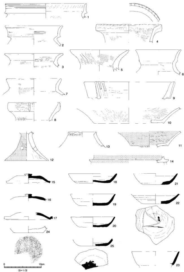
第16図 1区 SD08出土遺物 (S=1/3)
