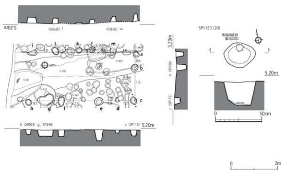
第262図 第97-3次調査区 掘立柱建物 遺構実測図1 (1/80)
