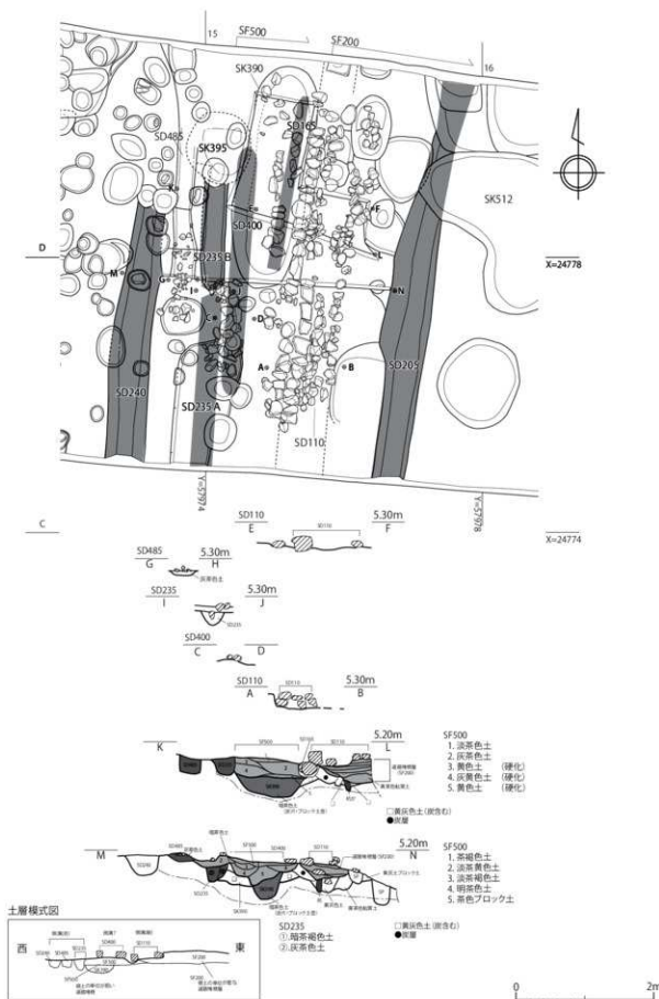
第278図 第97-3次調査区 SF200西側 遺構実測図 (1/60)
