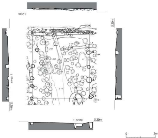
第263図 第97-3次調査区 掘立柱建物 遺構実測図2 (1/80)
