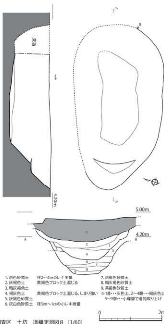
第229図 第97-2次調査区 土坑 遺構実測図8 (1/60)
