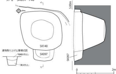
第224図 第97-2次調査区 土坑 遺構実測図3 (1/60)
