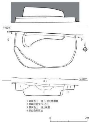
第222図 第97-2次調査区 土坑 遺構実測図1 (1/60)
