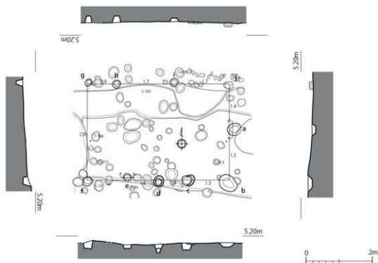
第265図 第97-3次調査区 掘立柱建物 遺構実測図4 (1/80)
