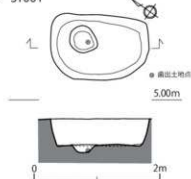
第230図 第97-2次調査区 土坑墓 遺構実測図 (1/60)
