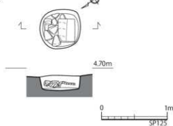
第231図 第97-2次調査区 柱穴 遺構実測図 (1/40)
