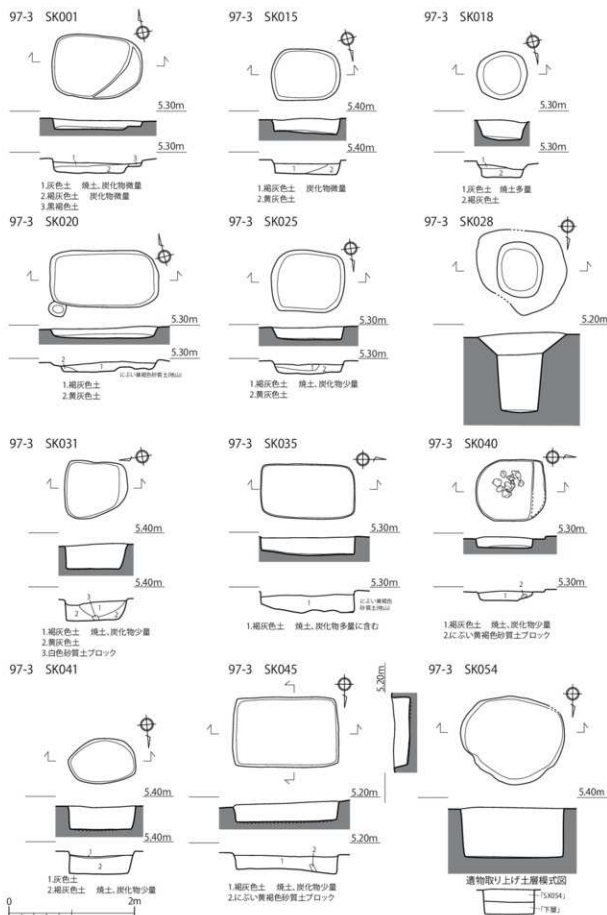
第269図 第97-3次調査区 土坑 遺構実測図1 (1/60)
