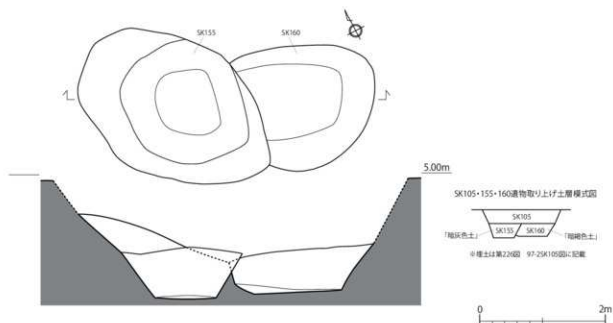
第227図 第97-2次調査区 土坑 遺構実測図6 (1/60)
