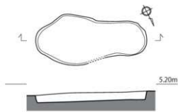
第271図 第97-3次調査区 土坑 遺構実測図3 (1/60)
