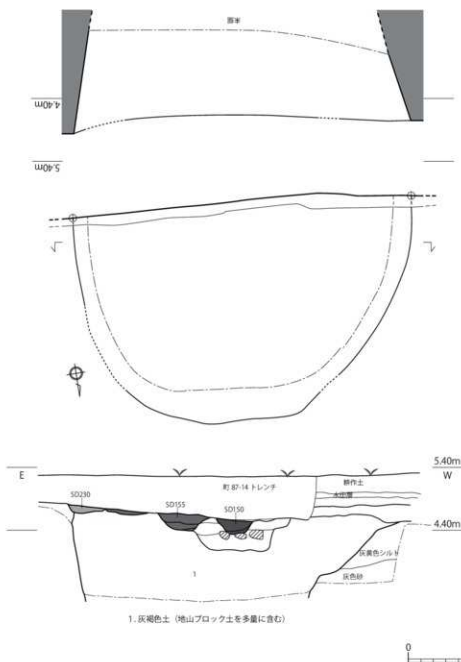
第 268 図 第 97-3 次調査区 井戸跡 遺構実測図 (1/60)
