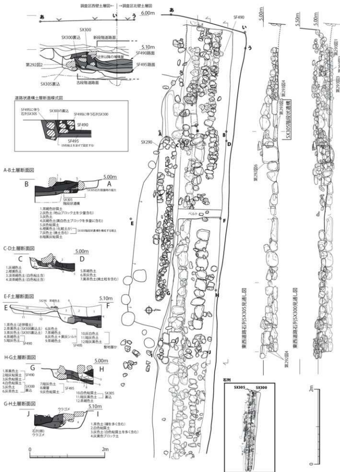
第280図 町97-3 調査区 SF490 遺構実測図 (1/50)
