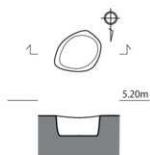
第276図 第97-3次調査区 柱穴 遺構実測図 (1/40)
