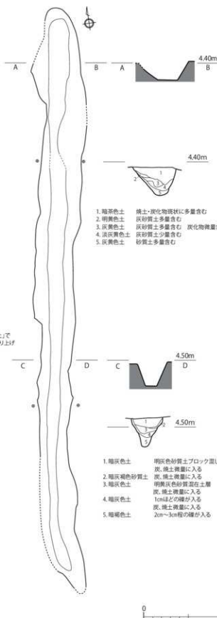
第156図 第97-1E次調査区 道路状道構 道構実測図1 (1/60)
