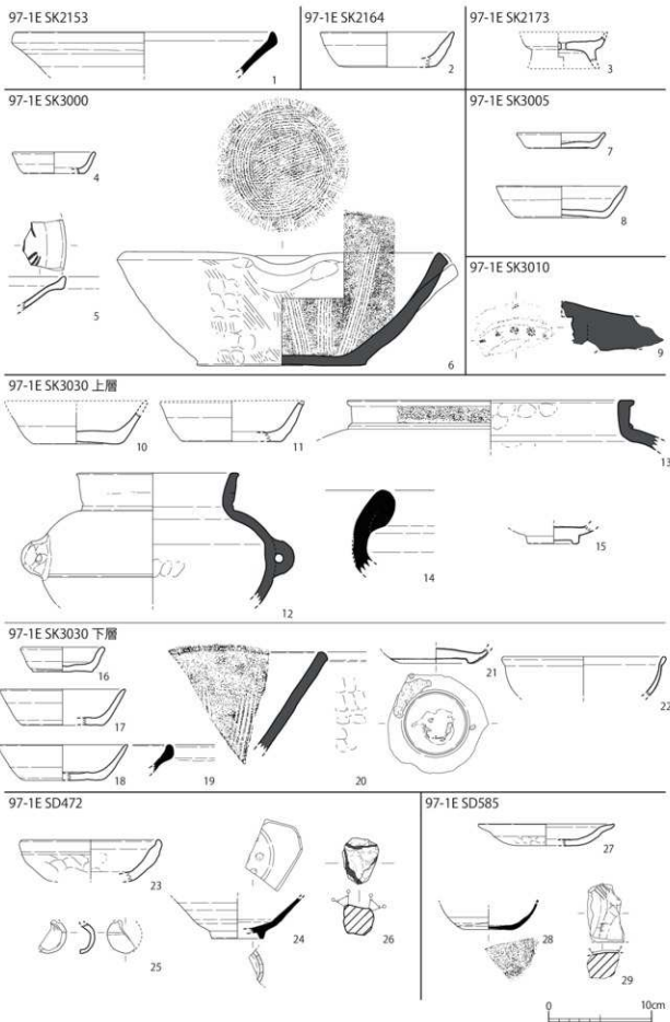
第192図 第97-1E次調査区 遺物実測図33 (1/4)
