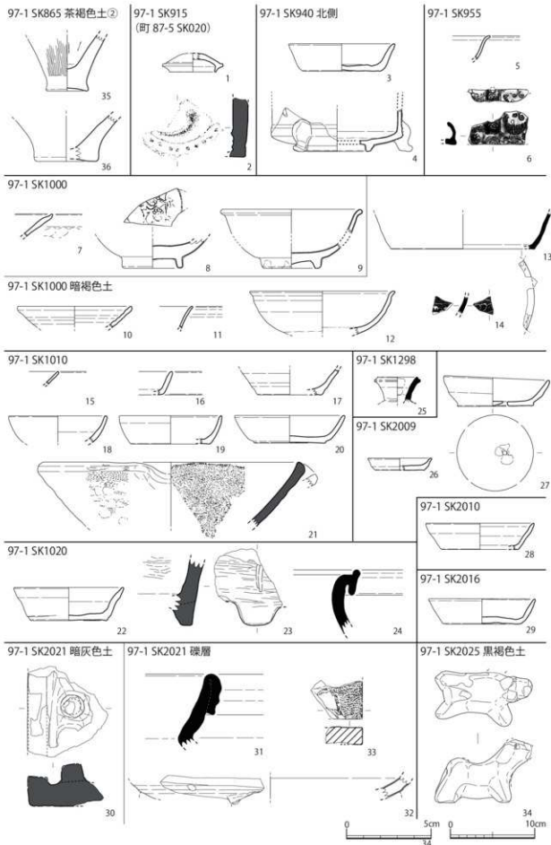
第 79 図 第 97-1 次調査区 遺物実測図 20 (1/2・1/4)
