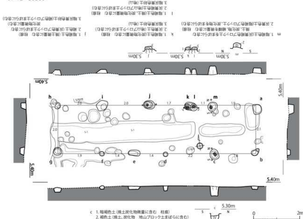
第 112 図 第 97-1E 次調査区 掘立柱建物 遺構実測図 4 (1/80)
