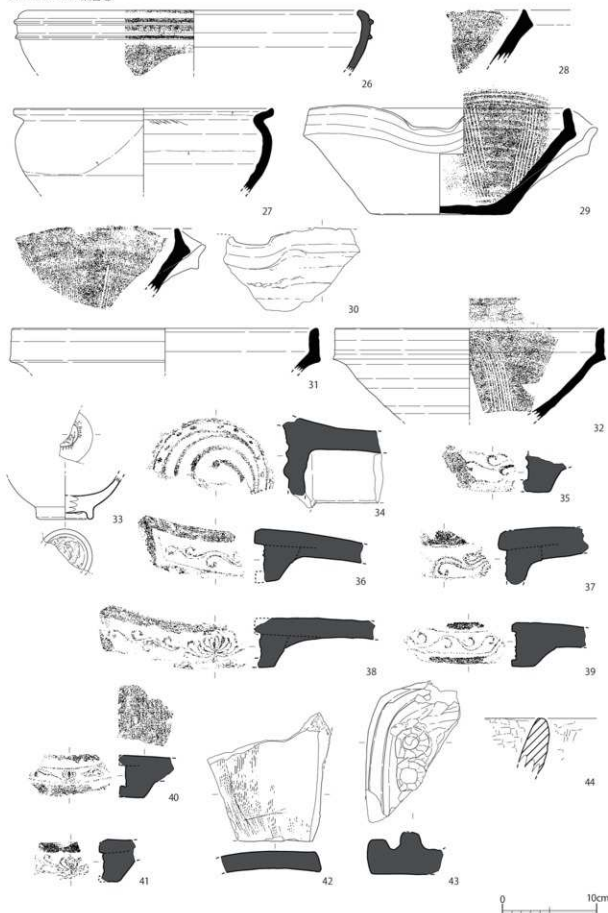
第 174 图 第 97-1E 次調査区 遺物実測図 15 (1/4)
