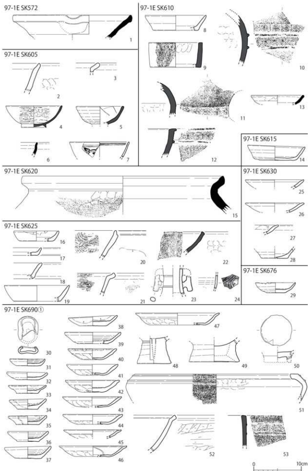
第181図 第97-1E次調査区 遺物実測図22 (1/4)
