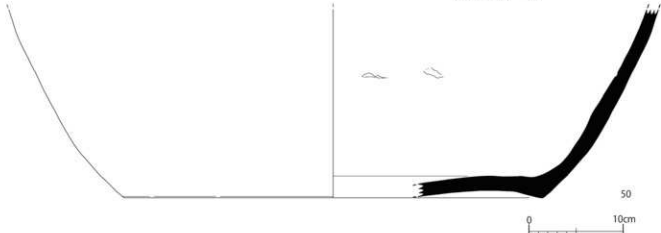
第193図 第97-1E次調査区 遺物実測図 34 (1/4)
