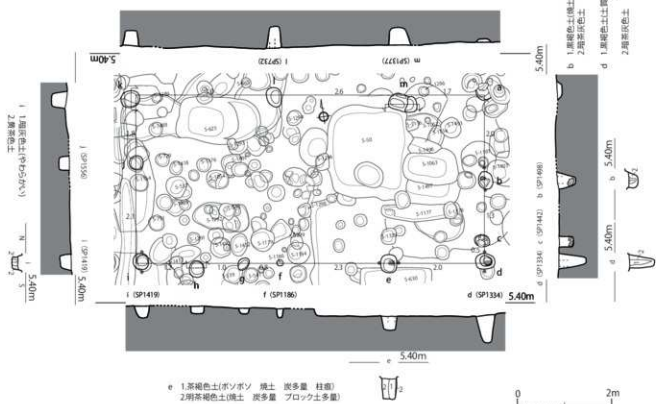
第123図 第97-1E次調査区 掘立柱建物 遺構実測図 15 (1/80)
