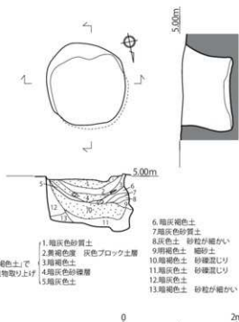
第40図 第97-1次調査区 土坑 遺構実測図 13 (1/60)
