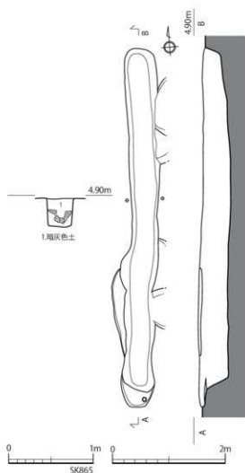
第43図 第97-1次調査区 土坑 遺構実測図 16 (1/40・1/60)
