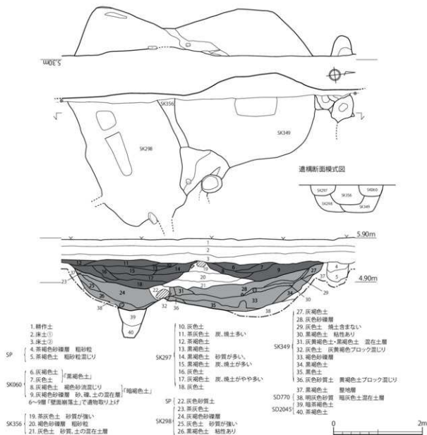
第31図 第97-1次調査区 土坑 遺構実測図4 (1/60)
