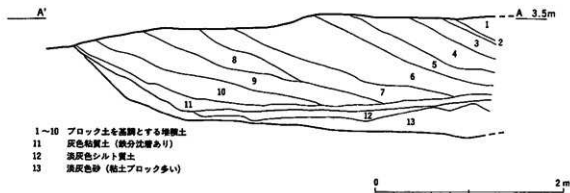
第11図 土層跡 (SX035) 土層図 (S=1/40)
