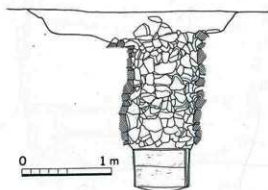
井戸実測図
