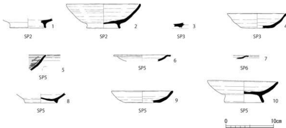
図16 手原遺跡 出土遺物実測図
