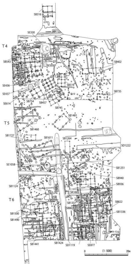
T4・T5・T6遺構平面図
