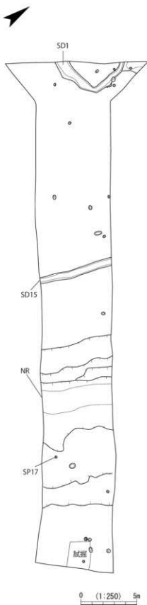
遺構平面図
