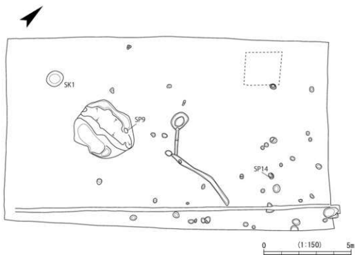
遺構平面図
