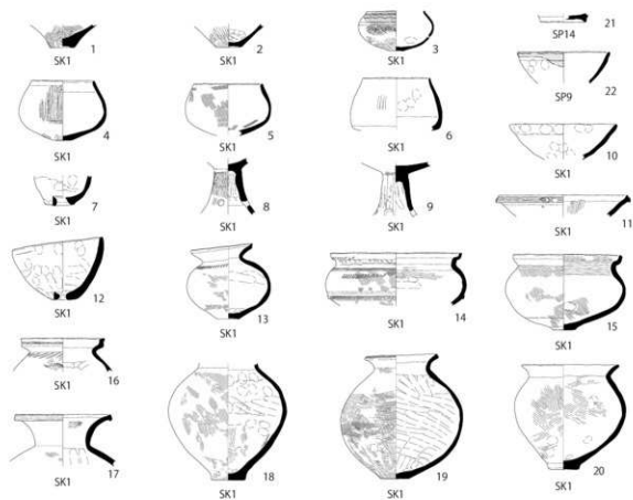
出土遺物実測図
