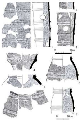
NR1北西肩口SD出土埴輪実測図
