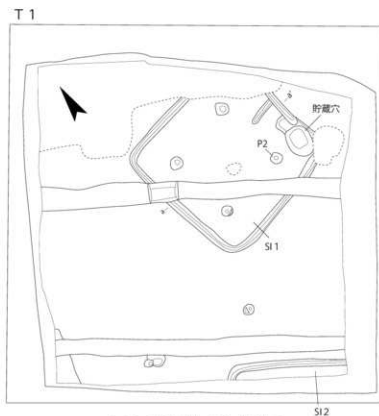
図8 高野遺跡 T1 遺構図
