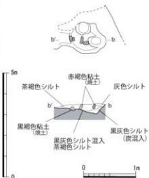
図11 高野遺跡 T2 SI 1 詳細図・断面図
