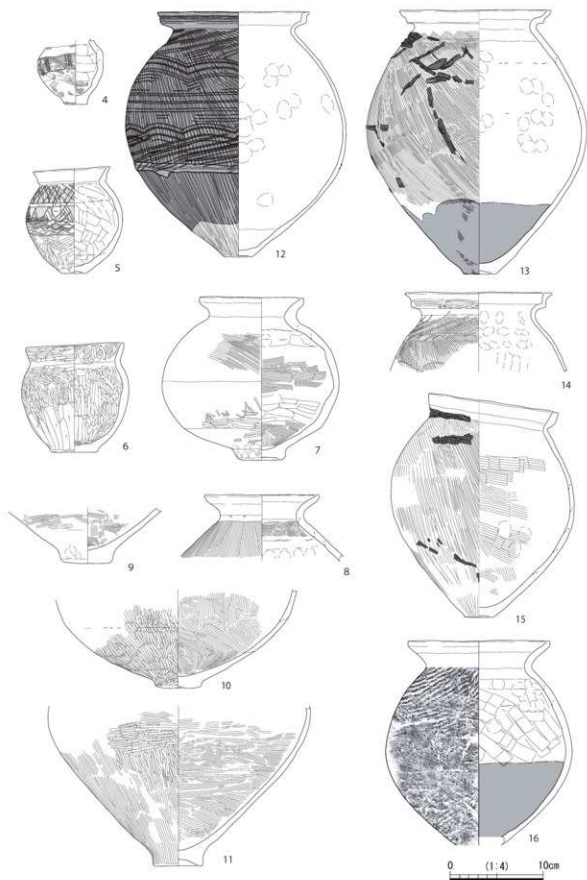
T11 SE2277出土遺物実測図
