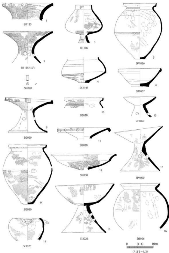
出土遺物実測図
