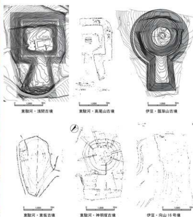
第72図 伊豆・東駿河における前期古墳測量図
