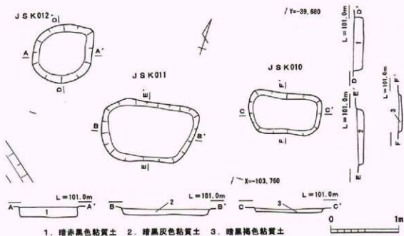
第108図 土坑 J S K 010・011・012 平・断面図
