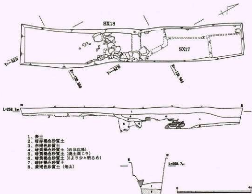
第21図 第10トレンチ実測図
