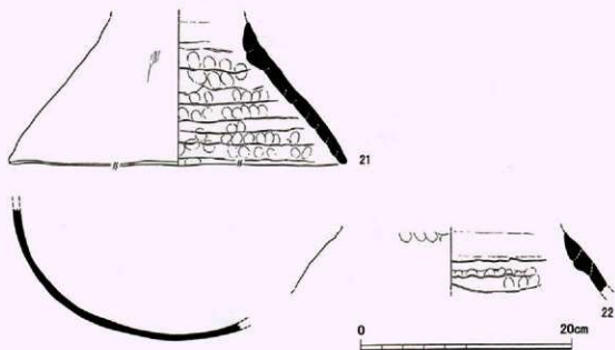
第88図 時塚1号墳出土埴輪実測図(3)
