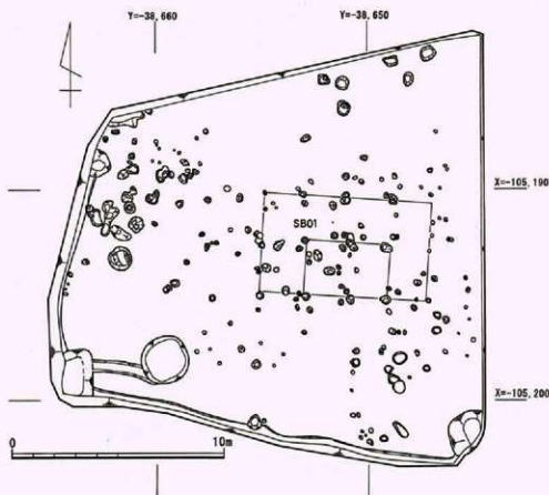
第124図 12トレンチ平面図
