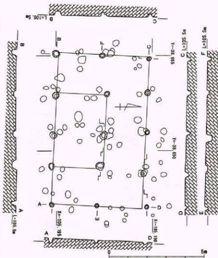
第125図 12トレンチ掘立柱建物跡実測図
