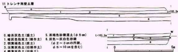
第123図 11トレンチ土層図
