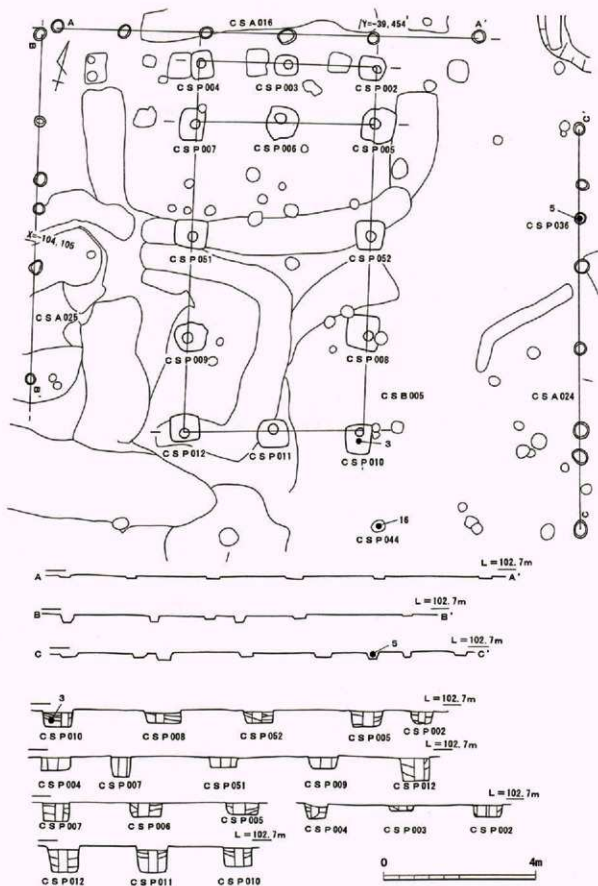
第54図 CSB005、CSA025・016・024実測図
