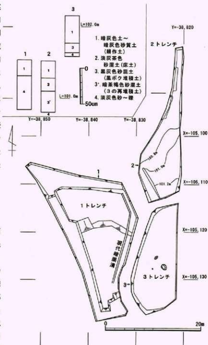
第115図 1～3トレンチ平面図、土層柱状図
