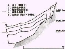
第17図 第7トレンチ土層断面図
