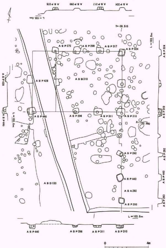
第53図 ASB310、ASA292実測図
