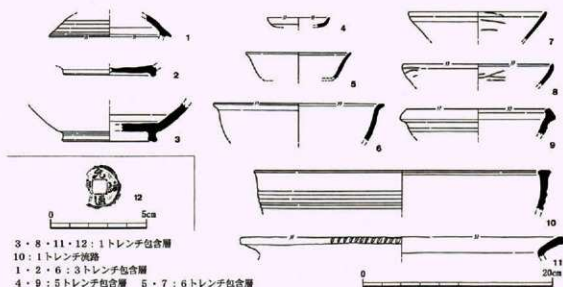
第5図 出土遺物実測図
