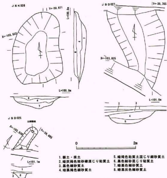
第110図 J-2トレンチ溝JSK025・027、土坑JSK026平・断面図
