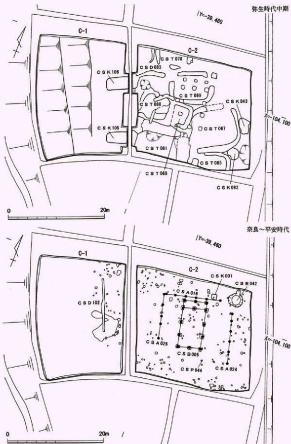
第6図 C地区(第6次)遺構配置図
