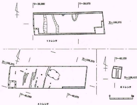
第3図 1・4・6トレンチ平面図
