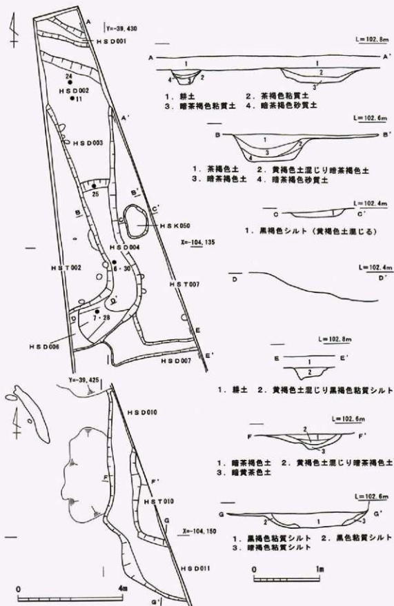
第20図 HST002・007・010実測図
