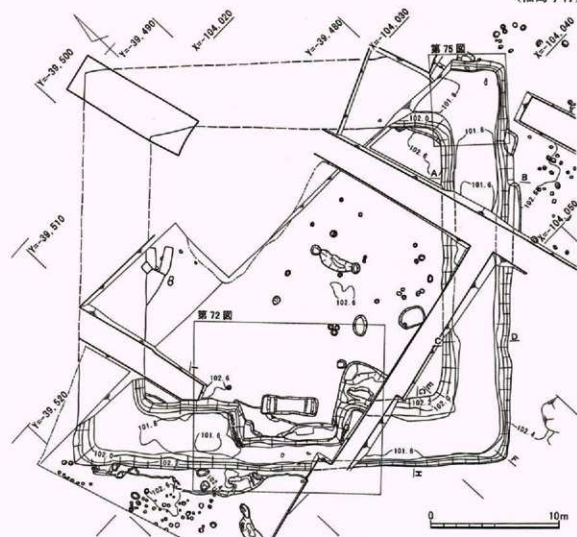
第70図 時塚1号墳平面図
