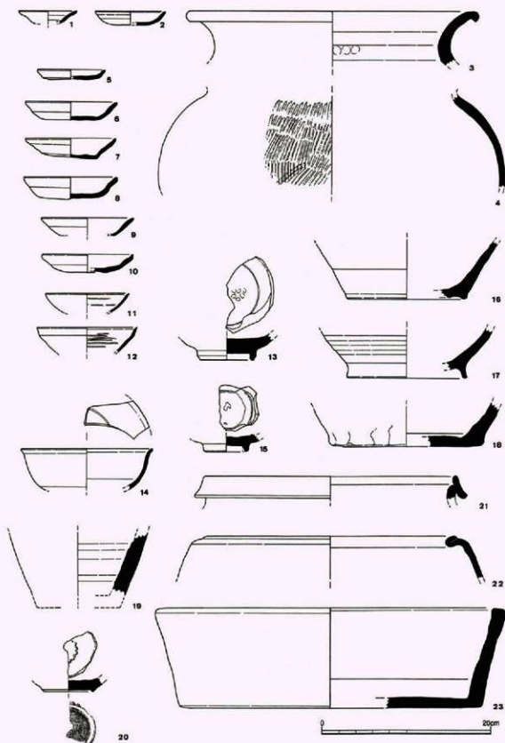
第22図 出土遺物実測図(1)
