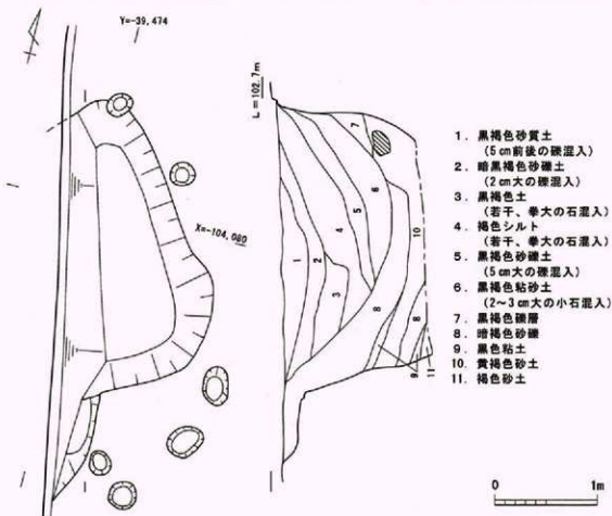
第65図 GSE492実測図
