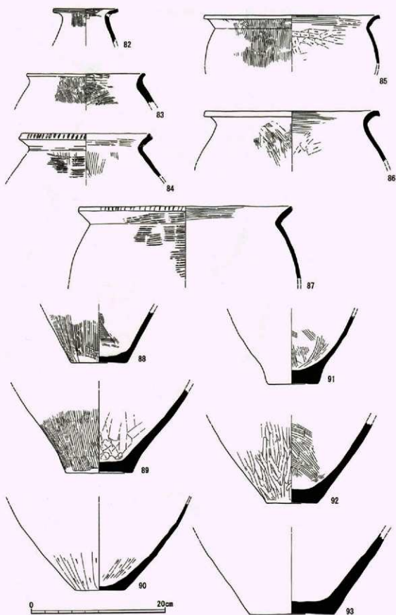
第38図 出土遺物実測図(弥生時代7 土坑出土遺物4)
