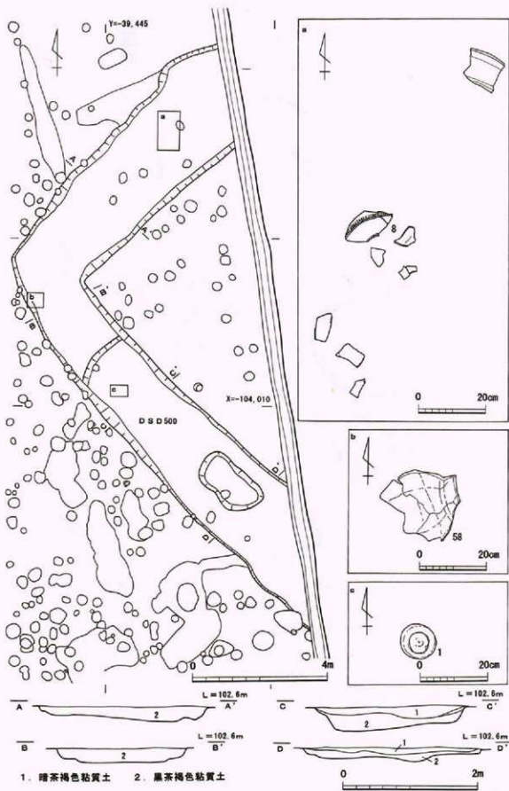
第100図 時塚2号墳実測図
