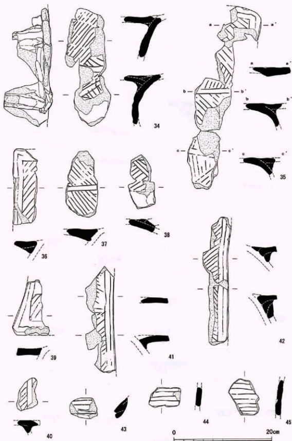
第91図 時塚1号墳出土地輪実測図(6)
