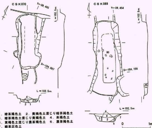
第19図 C S K 070・089実測図
