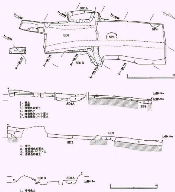
第7図 第1トレンチ実測図
