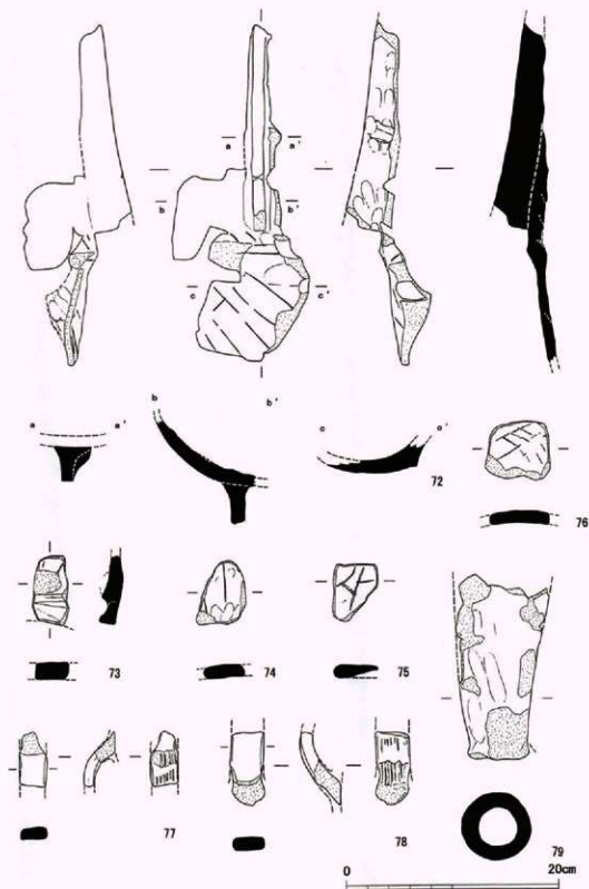
第94図 時塚1号墳出土埴輪実測図(9)
