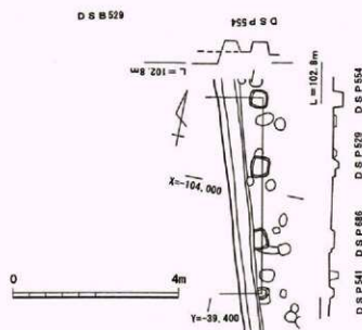
第55図 CSA052、DSB529実測図
