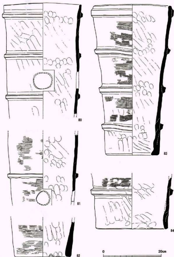
第95図 時塚1号墳出土形象埴輪円筒部実測図(10)
