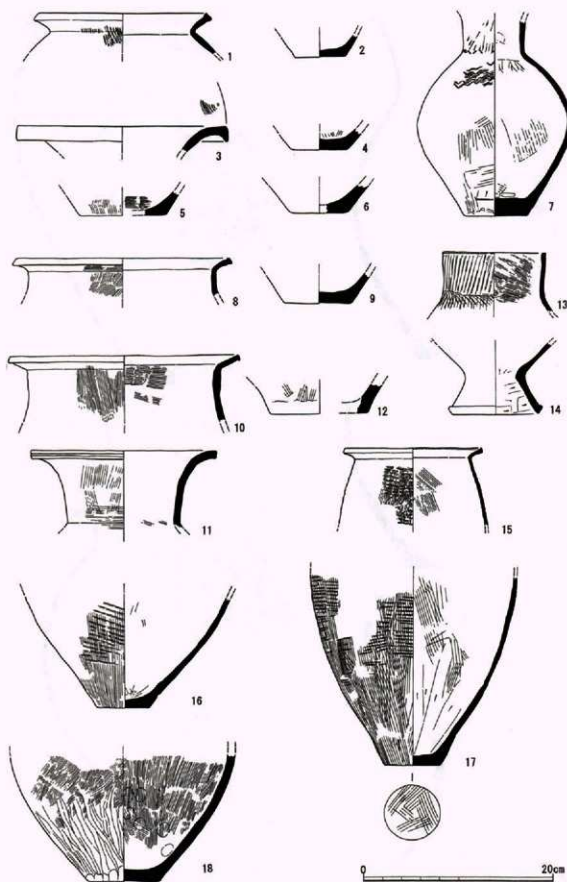
第111図 弥生土器実測図(方形周溝墓・溝・土坑)
