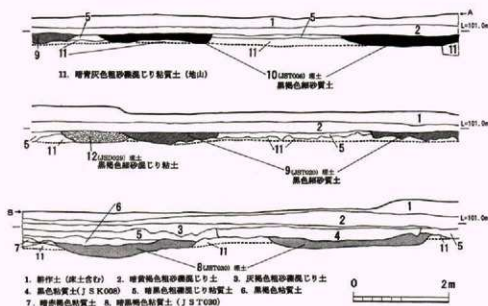
第102図 J地区土層図
