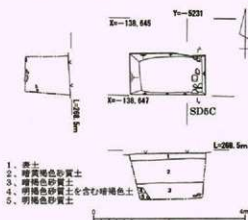
第9図 第3-3トレンチ実測図
