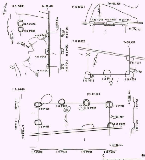
第57図 HSB041・021、ISB032・019実測図
