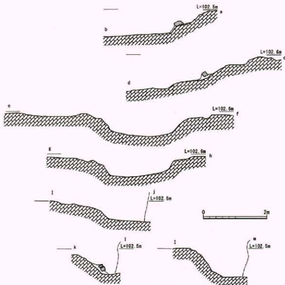
第74図 造出し部断面図
