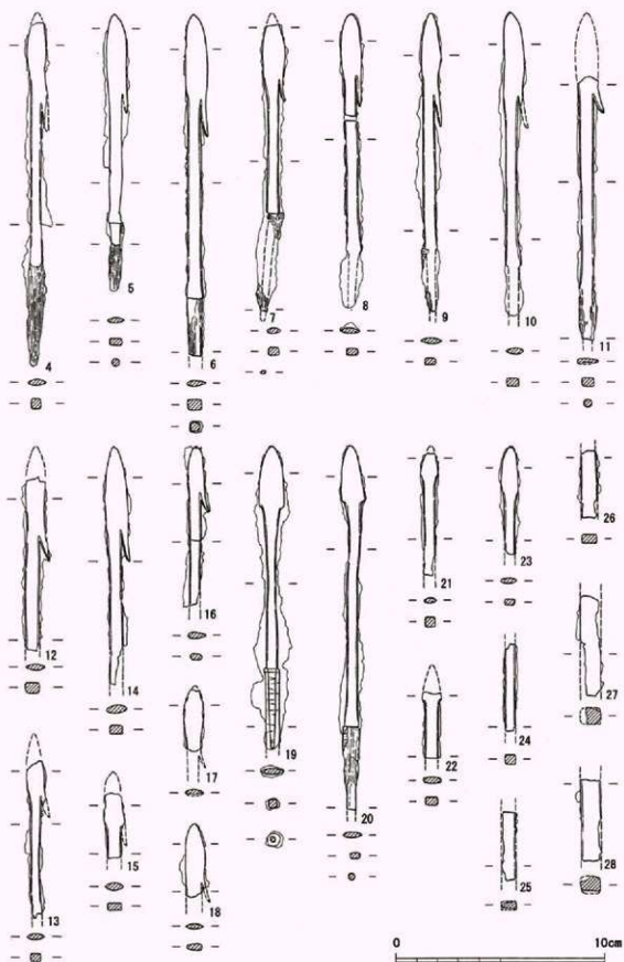
第80図 BSX033出土鉄器(2)
