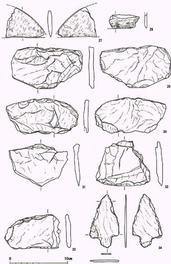
第46図 出土遺物実測図(磨製石器3)
