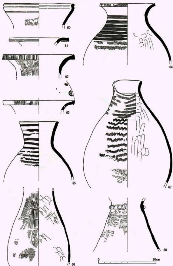
第36図 出土遺物実測図(弥生時代5 土坑出土遺物2)
