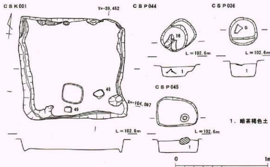
第61図 CSK001、CSP044・036・045実測図
