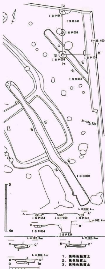
第58図 I S B 041、I S D 050・061実測図
