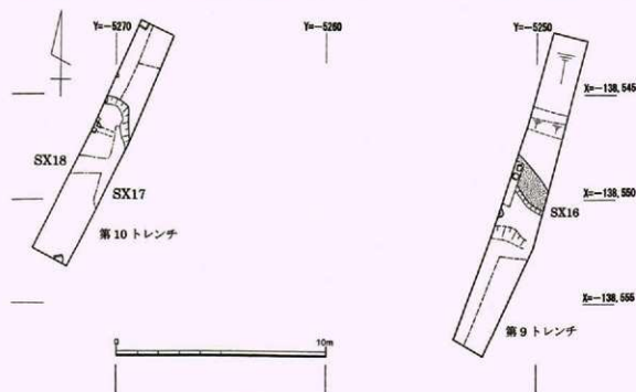
第20図 第9・10トレンチ実測図
