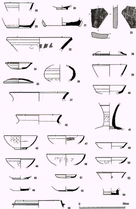
第129図 出土遺物実測図(弥生時代以降の土器2)
