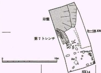
第18図 第7・8トレンチ実測図
