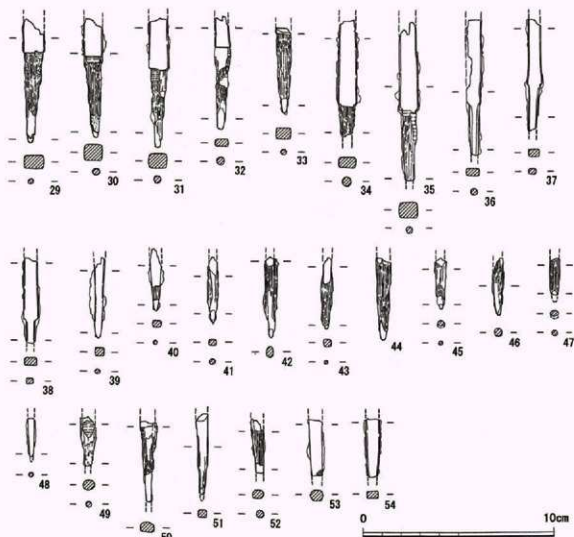
第81図 BSX033出土鉄器(3)
