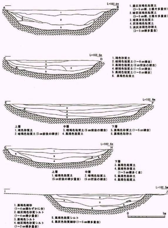
第71図 周溝内土層断面図
