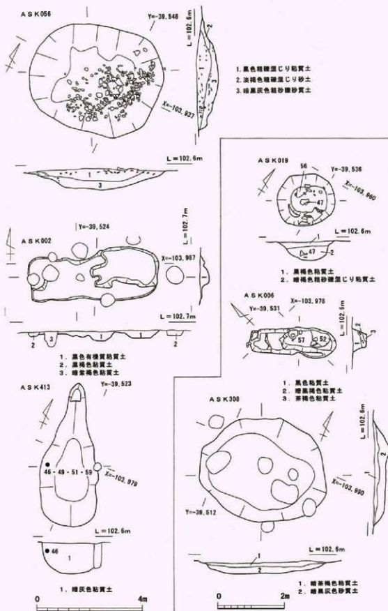
第25図 ASK056・002・413・019・006・308実測図
