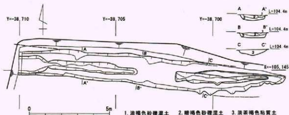
第121図 8トレンチ S D01平面図・土層図
