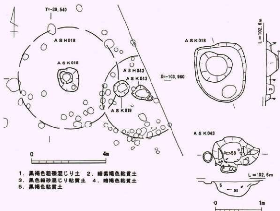
第13図 A S H018・043実測図
