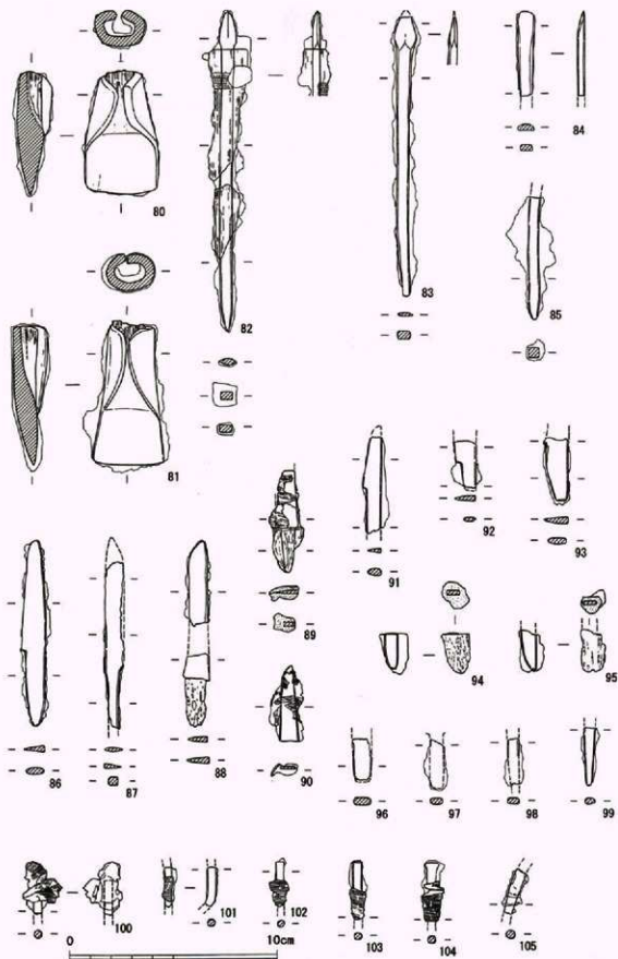
第85図 BSX033出土鉄器(7)
