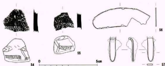
第99図 時塚1号墳周溝内出土土器実測図(3)
