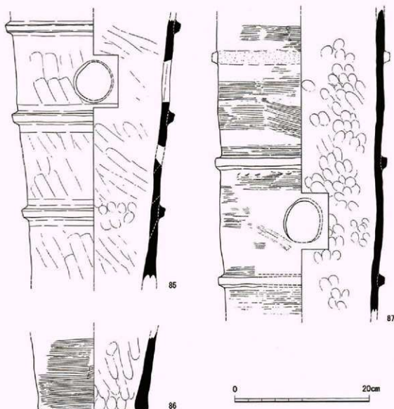
第96図 時塚1号墳出土形象埴輪円筒部実測図(11)
