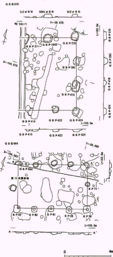
第56図 GSB370・644実測図
