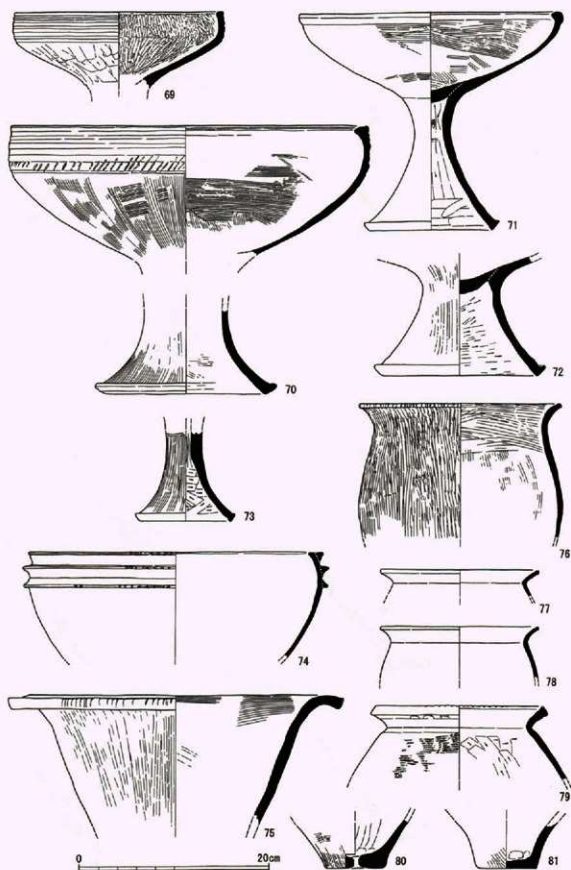
第37図 出土遺物実測図(弥生時代6 土坑出土遺物3)
