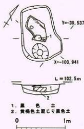
第11図 ASK344実測図および出土遺物実測図
