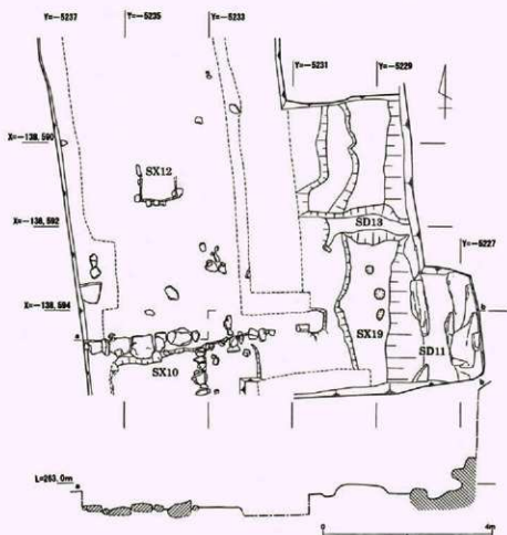
第16図 第6トレンチ南部実測図
