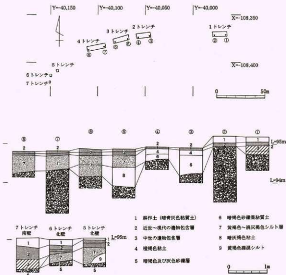
第4図 各トレンチ土層柱状図
