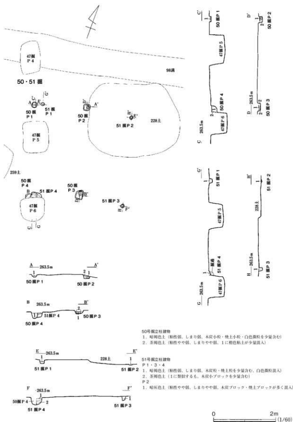
第42図 50・51号掘立柱建物
