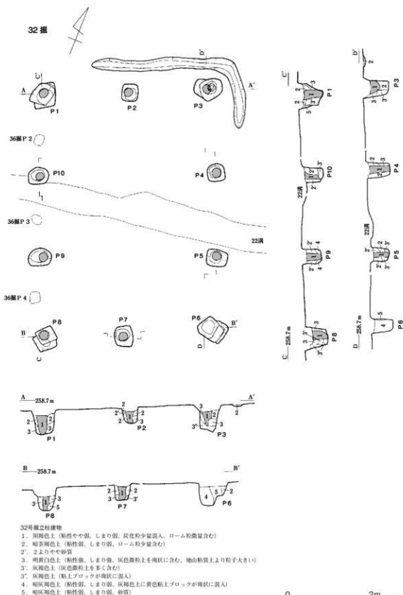
第25図 32号掘立柱建物
