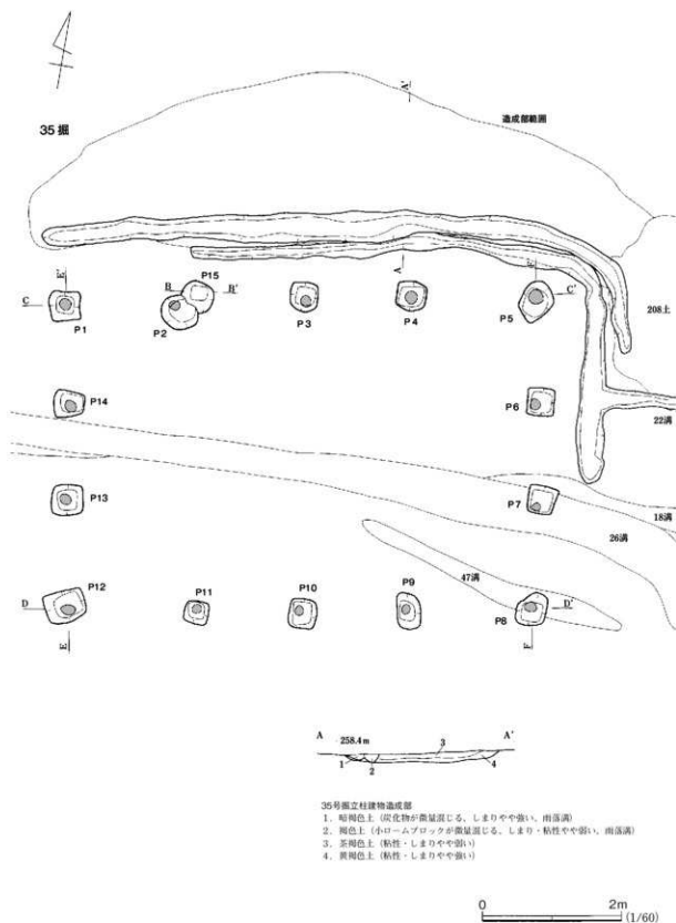
第27図 35号掘立柱建物 (1)
