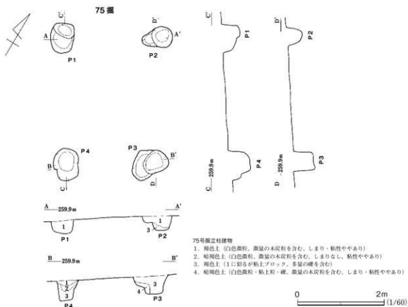
第64図 73・75号掘立柱建物
