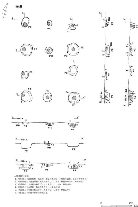
第37図 46号掘立柱建物
