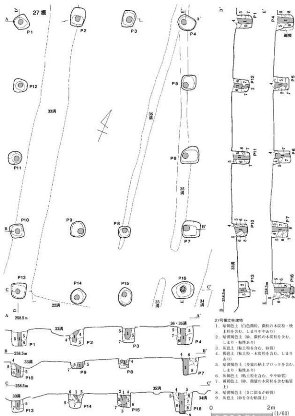
第21図 27号掘立柱建物
