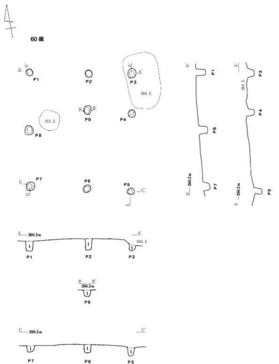
60号独立柱建物
