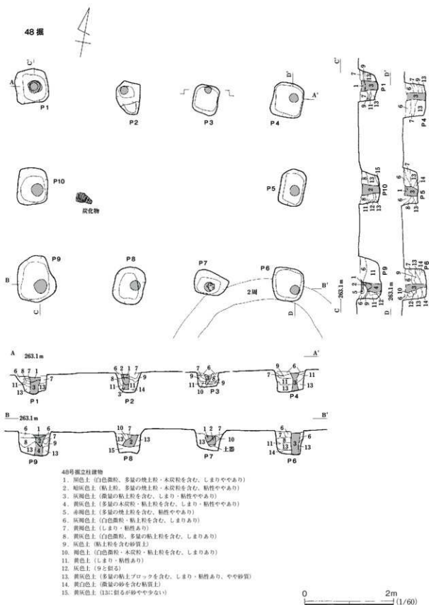
第40図 48号掘立柱建物
