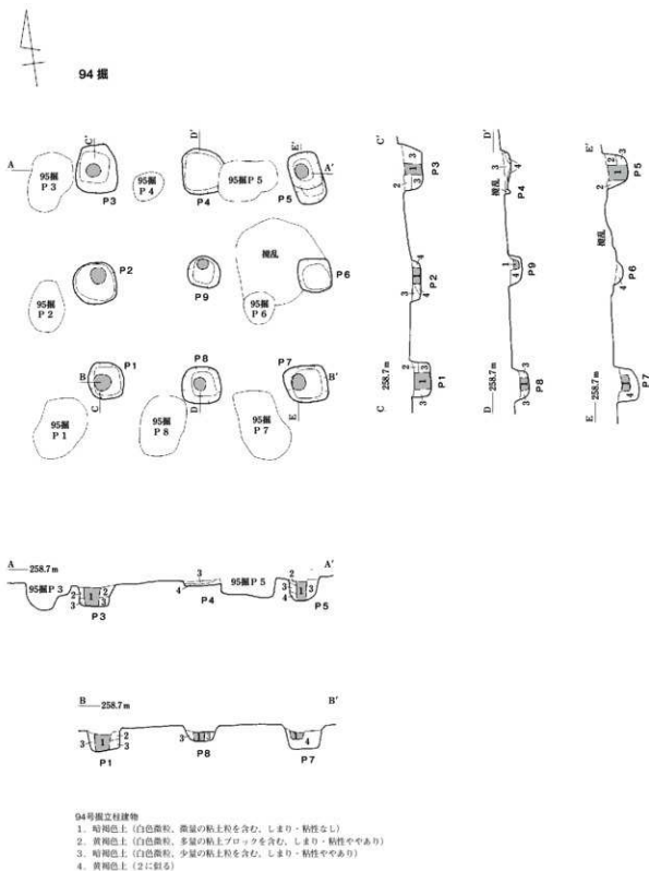
第87図 94号掘立柱建物
