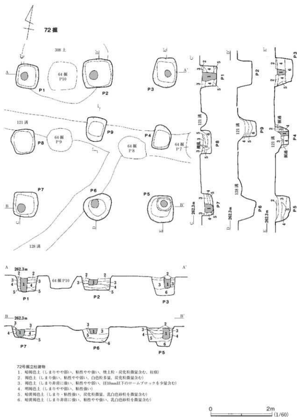
第63図 72号掘立柱建物
