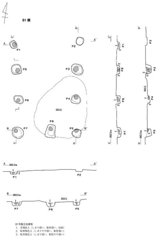
第73図 81号掘立柱建物
