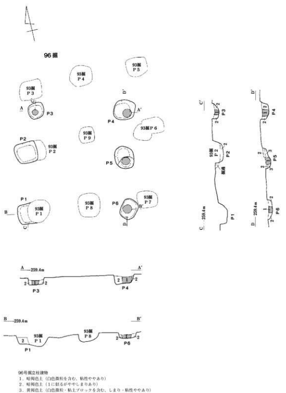
第89図 96号掘立柱建物
