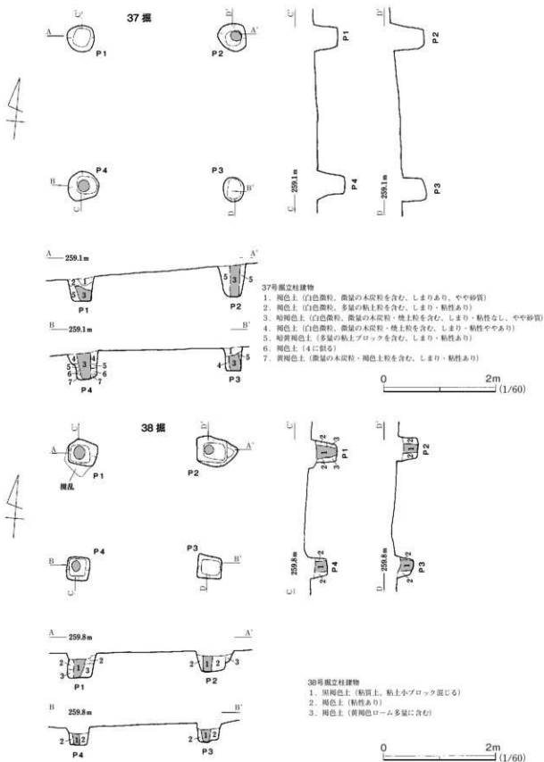
第29図 37・38号掘立柱建物
