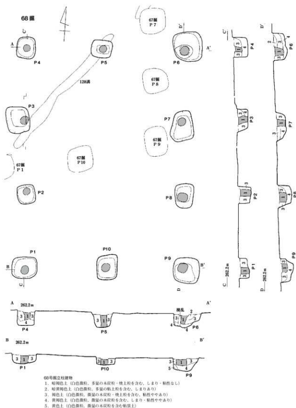
第59図 68号掘立柱建物
