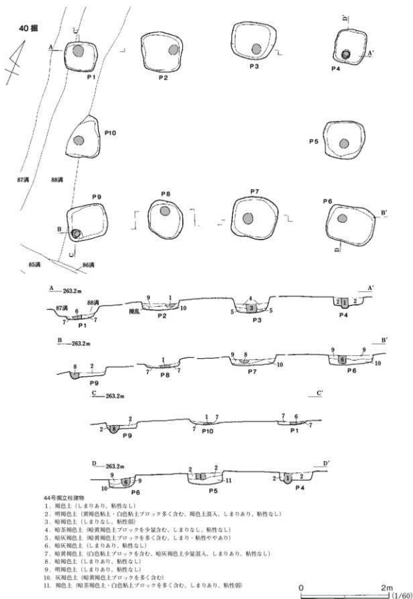
第35図 44号掘立柱建物
