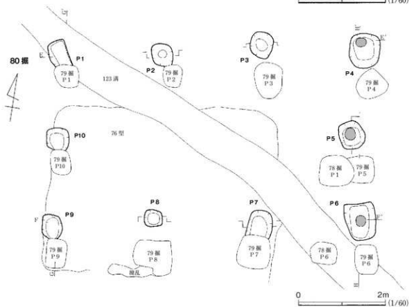
第70図 79・80号掘立柱建物 (1)
