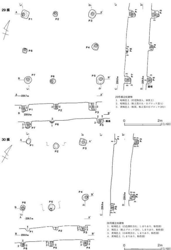
第23図 29・30号掘立柱建物
