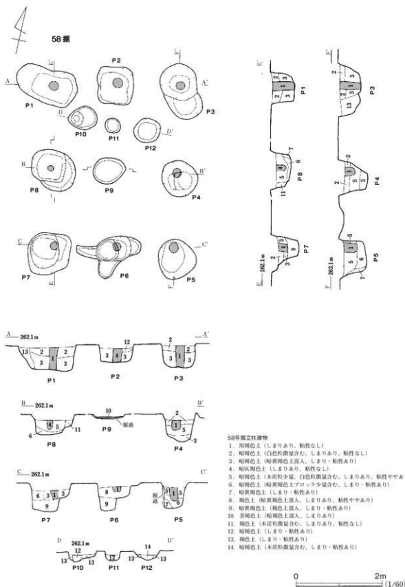
第49図 58号掘立柱建物
