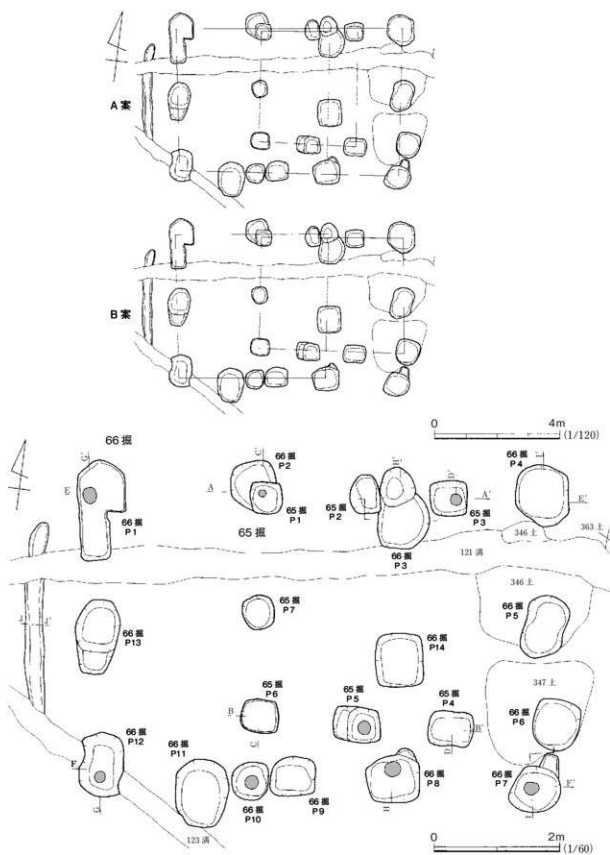
第56図 65・66号掘立柱建物 (1)
