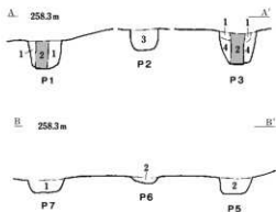
77号掘立柱建物
