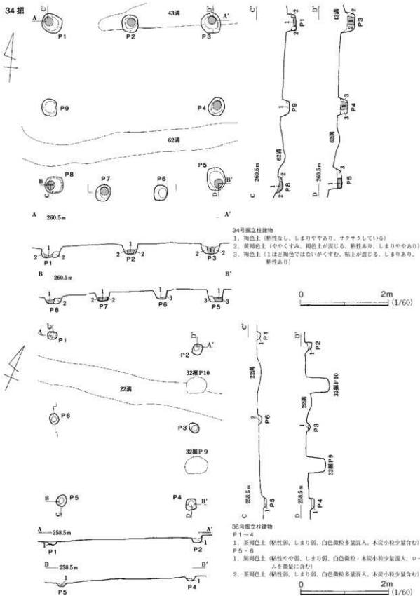
第26図 34・36号掘立柱建物
