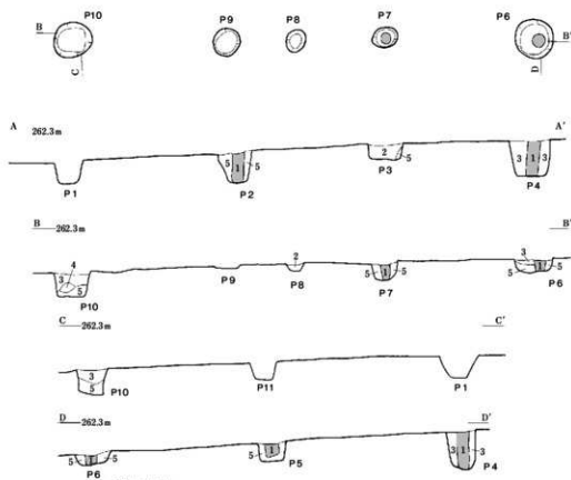
40号掘立柱建物
