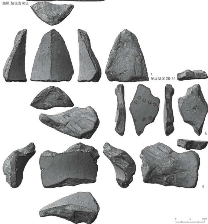
第209図 鵜尾 第1・2次、桜坂古窯址（3次元計測画像）
