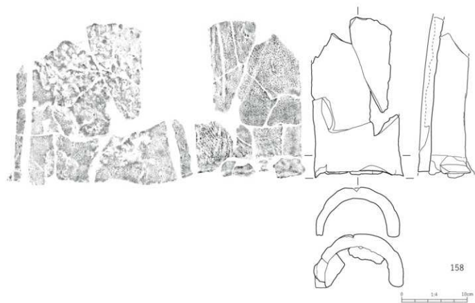
第166図 軒丸瓦接合丸瓦 粘土板桶巻づくりⅠ類
