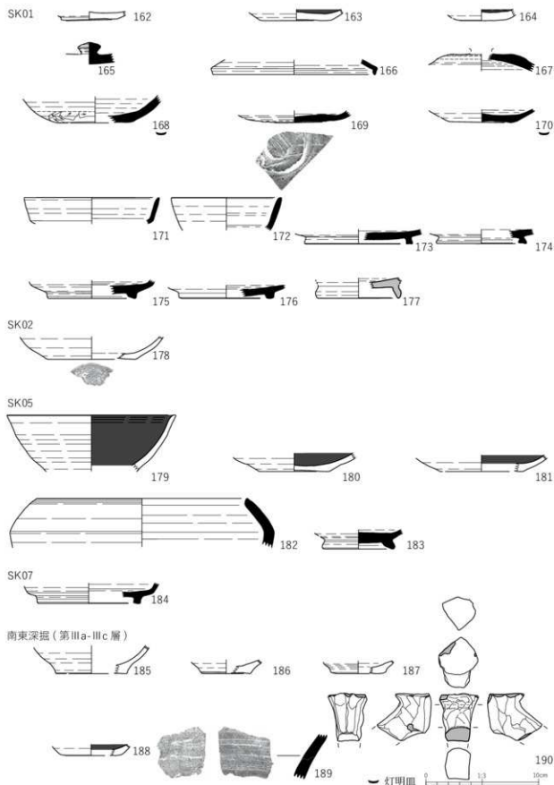
第219図 土器類 (SK01、SK02、SK05、SK07、南東深掘)
