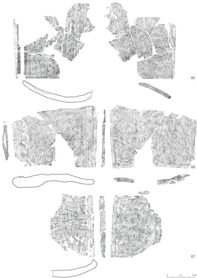
第182図 平瓦 粘土板桶巻づくりⅡ③類
