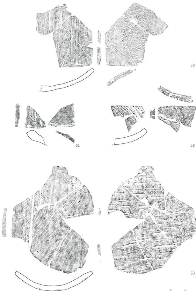
第178図 平瓦 粘土板桶巻づくりⅡ②類
