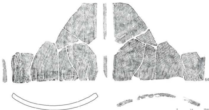
第181図 平瓦 粘土板桶巻づくりⅡ③類
