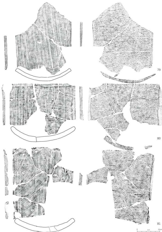
第185図 平瓦 粘土板桶巻づくりⅡ③類
