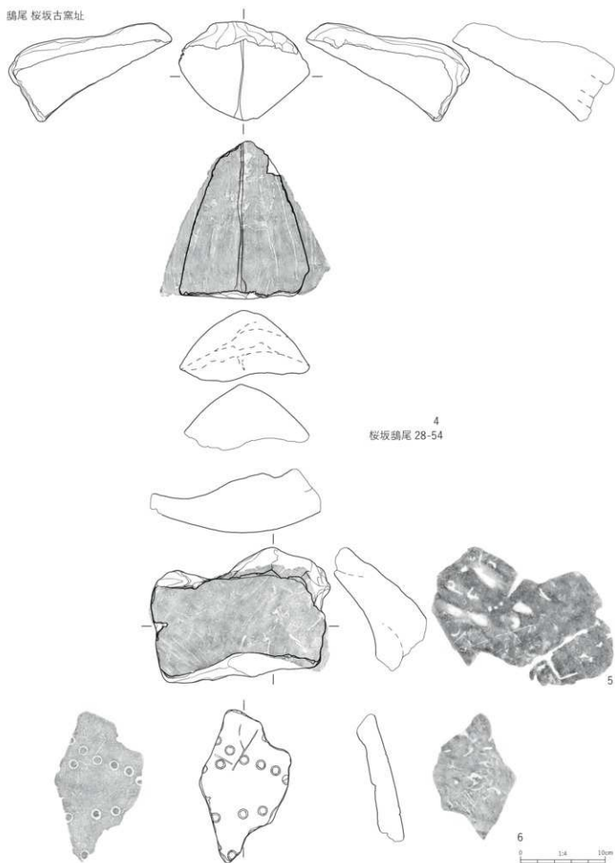
第208図 鷗尾 桜坂古窯址
