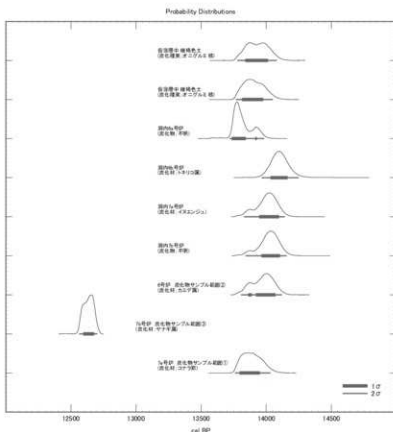
第 90 図 暦年較正結果 (1σ・2σ)
