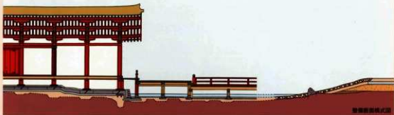
整備前断面模式図
