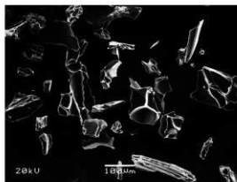
B-Tm。主としてバブルウォール型火山ガラス。下方に繊維状軽石型火山ガラス
