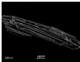
B-Tmの繊維状軽石型火山ガラス
