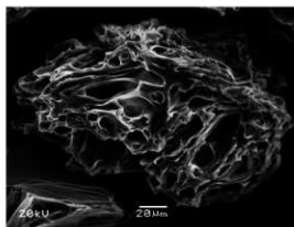
Ko-dの軽石型火山ガラス
