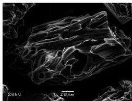
Ko-dの軽石型火山ガラス
