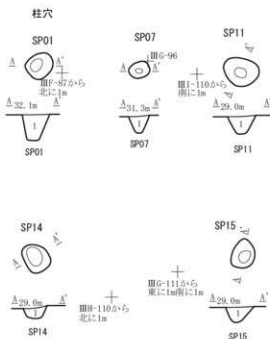
図8 掘立柱建物跡・柱穴
