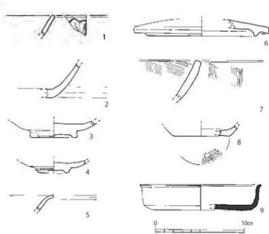
第61図 1号大溝出土土器・陶磁器実測図（1/3）
