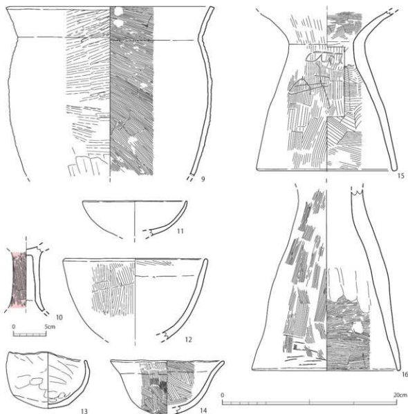
第16図 谷部出土土器実測図② (1/3、10・11は1/4)
