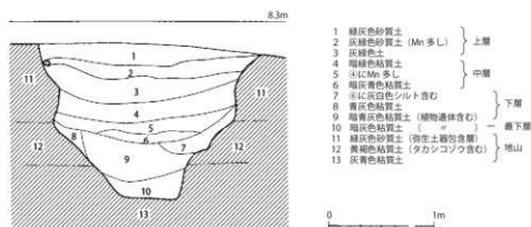
第39図 2号大溝土層実測図 (1/40)
