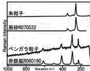
6 同赤色顔料のラマン分光スペクトル図（資料6） 朱からは辰砂を、ベンガラからは赤鉄鉱を同定した。比較資料はRRUFFより引用。
