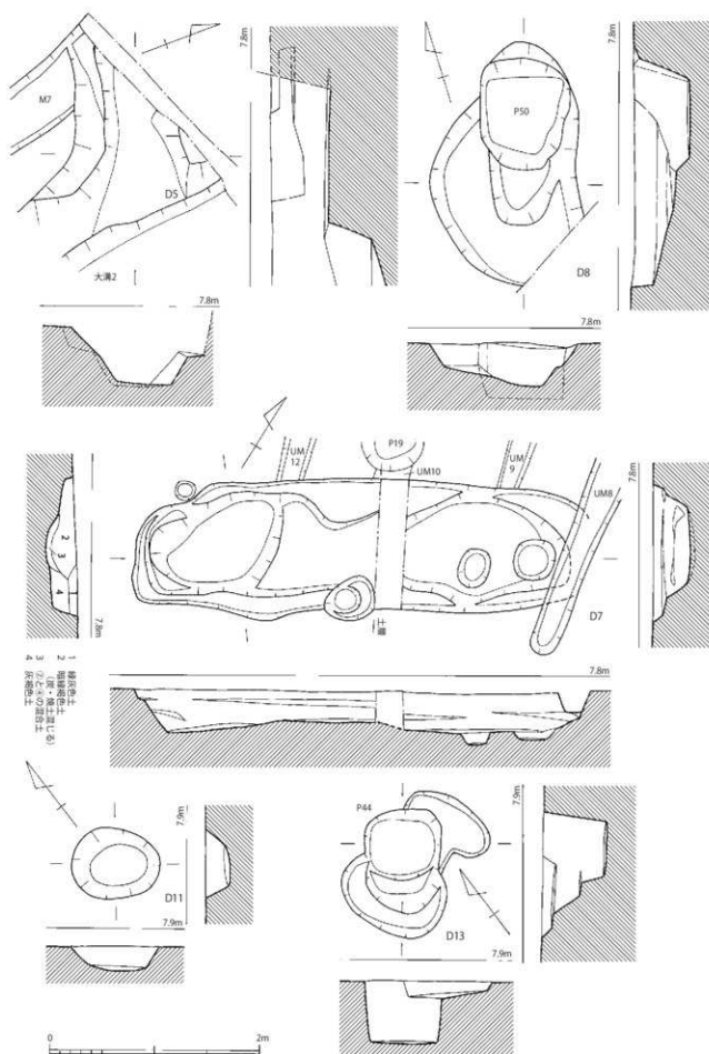
第32図 5・7・8・11・13号土坑実測図 (1/40)
