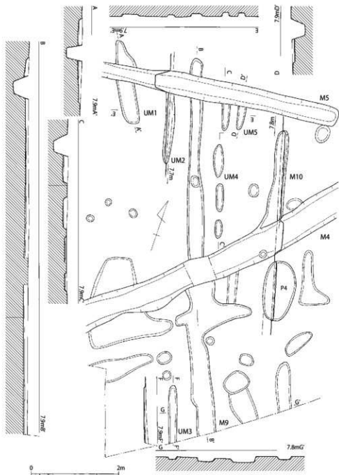
第82図 4・5・9・10号溝、1～5号縦溝実測図 (1/60)
