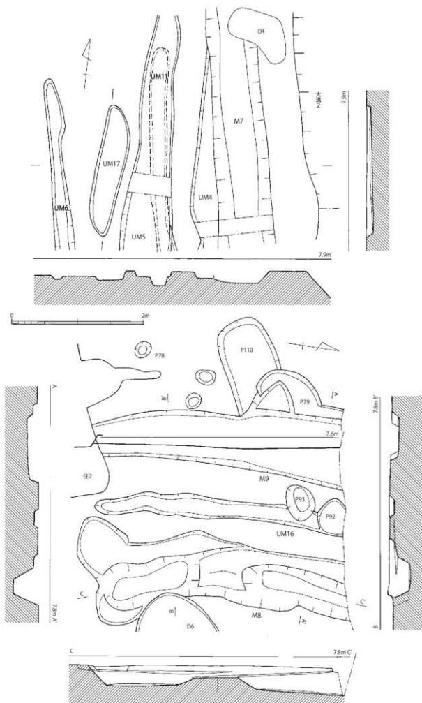
第44图 7~9号溝、4~6・11・16・17号畝溝実測図 (1/40)
