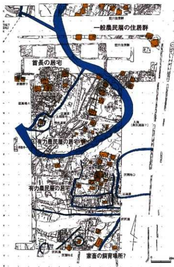
坂屋遺跡の集落構成図（6世紀末）
