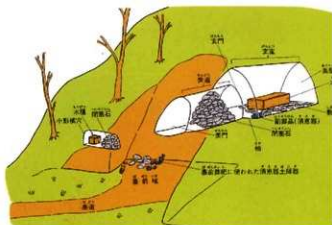
横穴墓の構造
