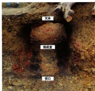
完掘された衛門坂4号窯
