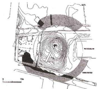
墳丘復原図
