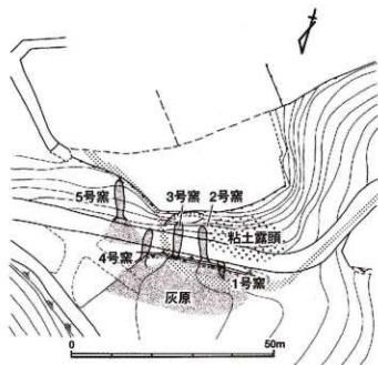
衛門坂古窯跡群配置図
