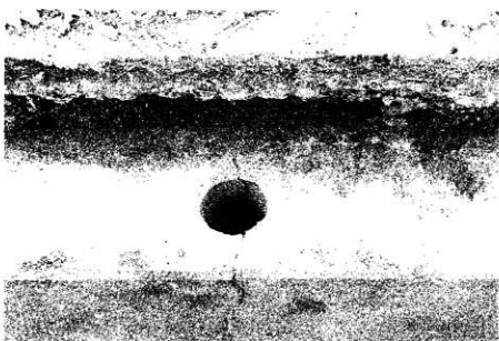
写真15-8 右基礎中心に建てられたと思われる丸太杭跡
