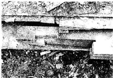
写真13-3 東側土台継手
