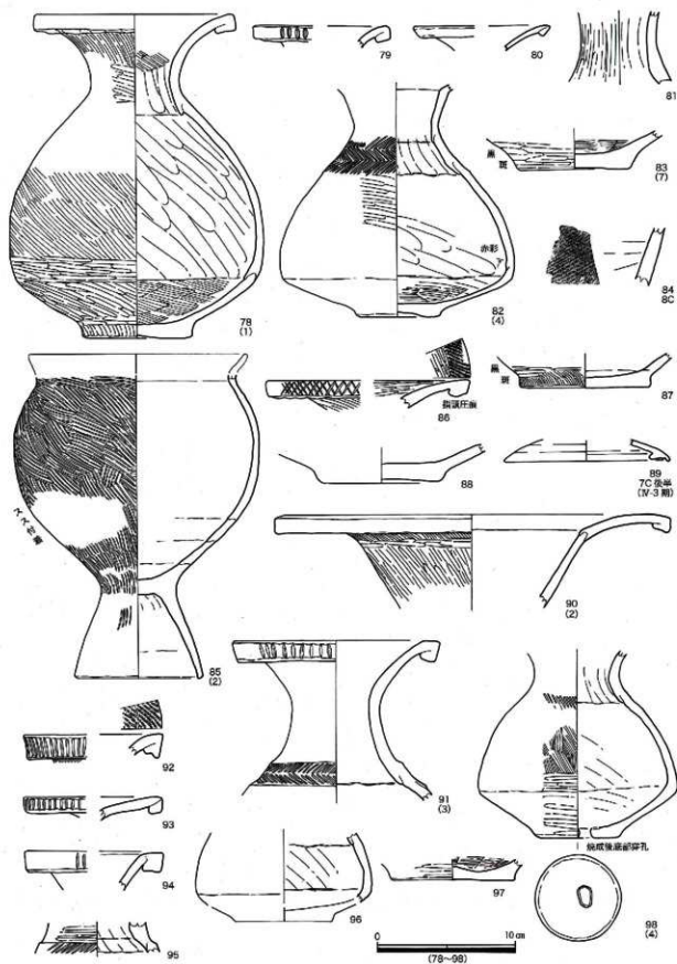
第82圖 第46・56次 土器実測図5
