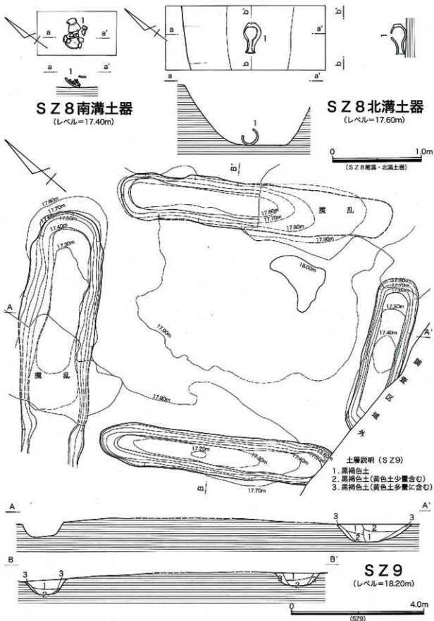
第55図 第46・56次 SZ8土器出土状況図、SZ9実測図
