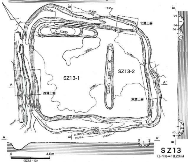
第57図 第46・56次 SZ12・13実測図
