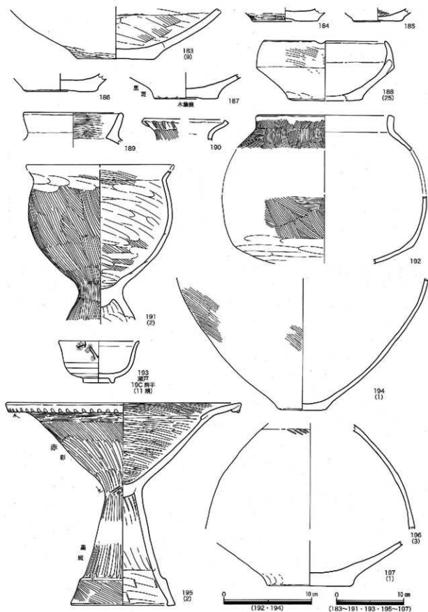
第91図 第46・56次 土器実測図14
