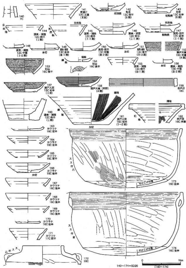
第38図 第44・45次 土器実測図5
