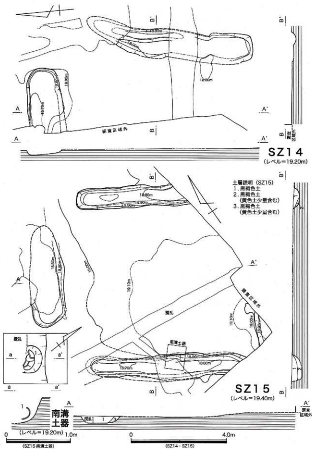
第9図 第38～40・48次 SZ14・15 実測図
