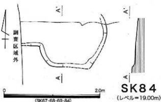
第31図 第44・45次 SK67～70・79・84 実測図
