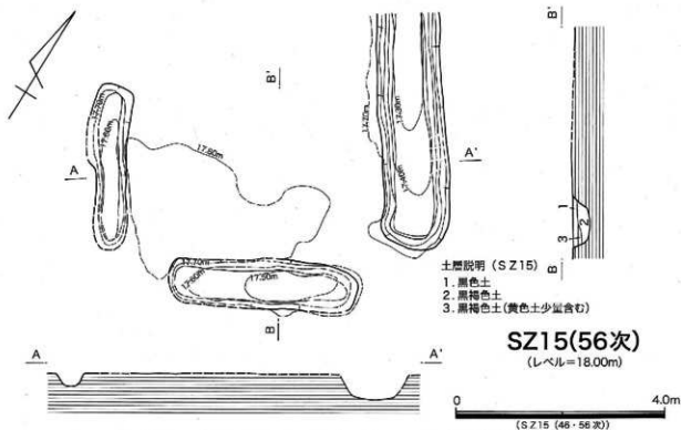
第63図 第46・56次 SZ15 (46次)・SZ15 (56次) 実測図
