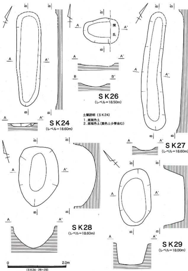
第74図 第46・56次 SK24・26～29実測図
