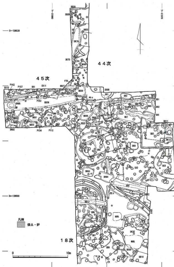
第27図 第44・45次 発掘調査区全体図
