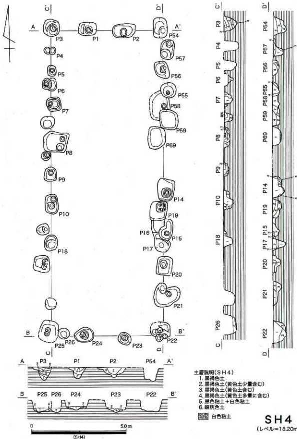
第47図 第46・56次 SH4実測図
