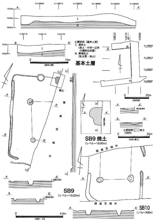
第21図 第41～43次 基本土層図、SB9・10実測図
