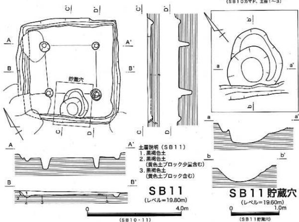
第4図 第38~40・48次 SB10・11 実測図
