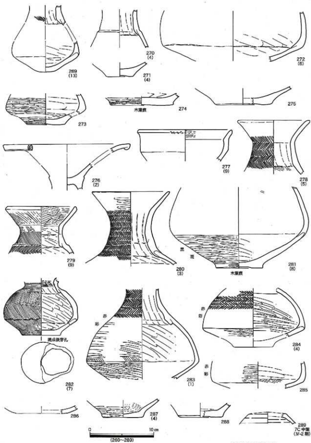
第97図 第46・56次 土器実測図20
